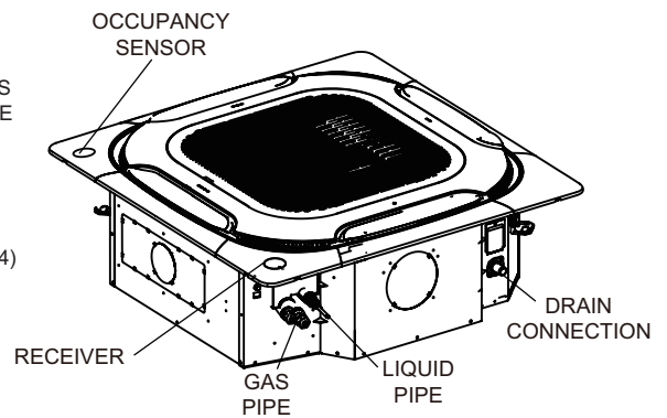
BOTTOM (PANEL) VIEW
