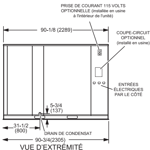
VUE D'EXTRÉMITÉ
