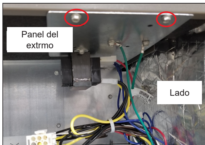
FIGURA 19. Panel de control reubicado al panel extremo (configuración horizontal derecha)
