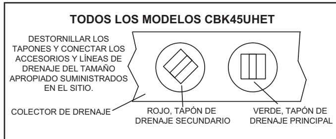
FIGURA 14. Conexiones de las líneas de drenaje
