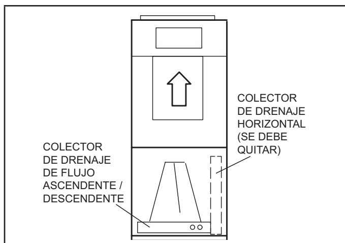
FIGURA 3. Configuración de flujo ascendente APLICACIONES HORIZONTALES
