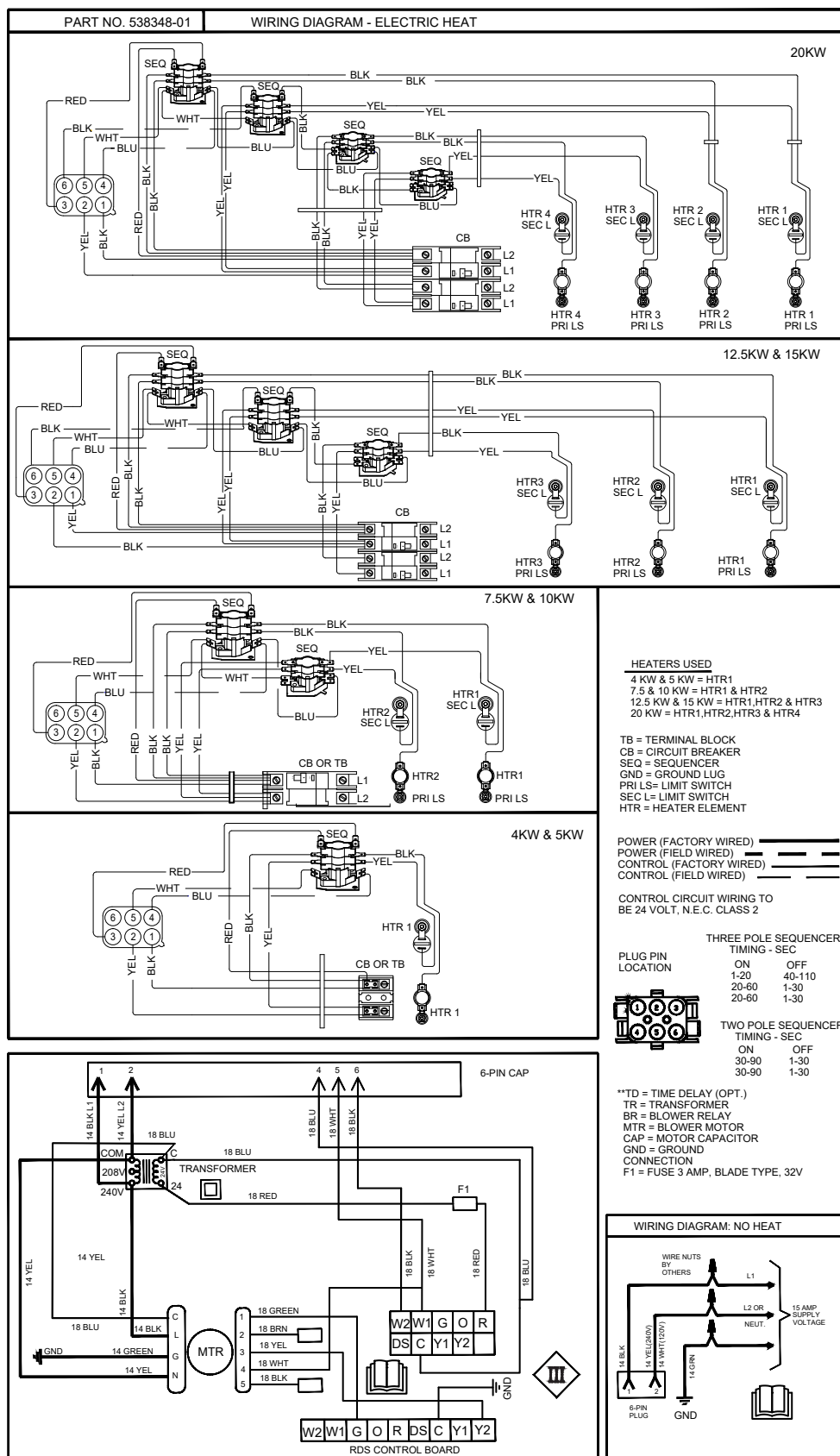
FIGURA 1. Diagrama de cableado típico – Unidad de manejo de aire CBK45UHET con calefacción eléctrica – CT
