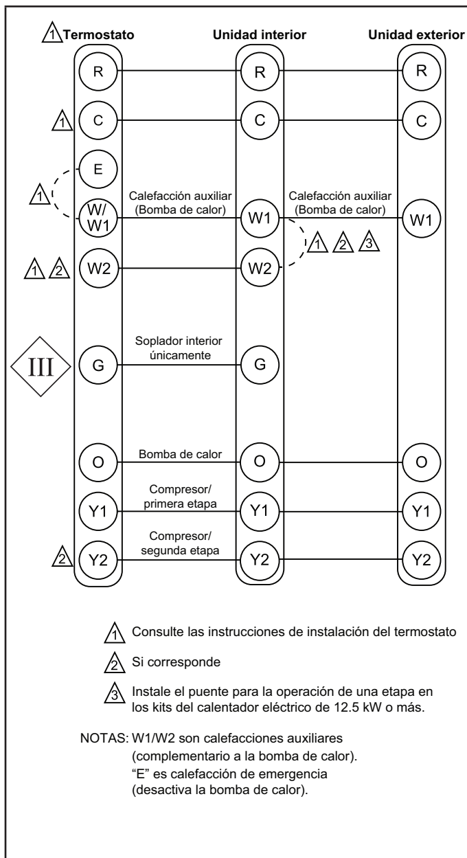
FIGURA 2. Designaciones del termostato – Sin comunicación
