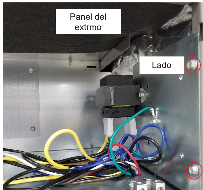
FIGURA 17. Conexiones eléctricas (configuración de flujo ascendente)
