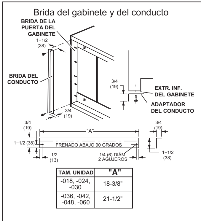
FIGURA 15. Brida del gabinete y del conducto
