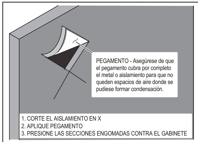
FIGURA 21. Reparación del aislamiento
