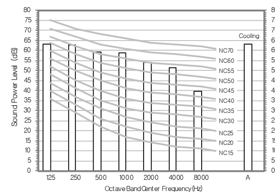
4) MMD036S6-1P
