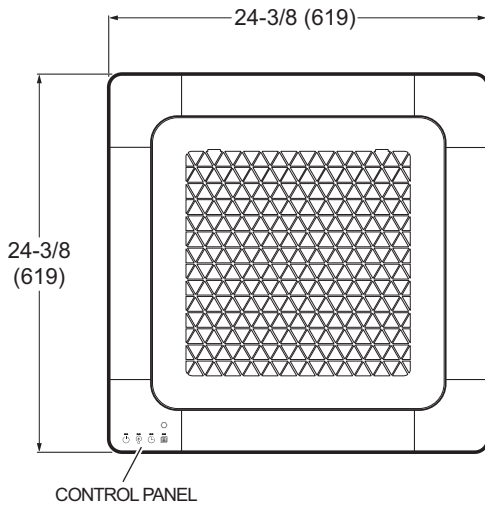
BOTTOM VIEW (Panel)
