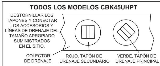
FIGURA 12. Conexiones de las líneas de drenaje
