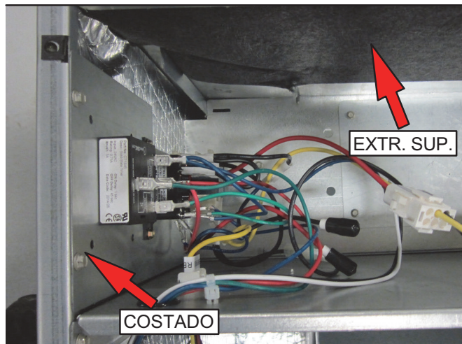
FIGURA 15. Conexiones eléctricas (configuración de flujo ascendente)
