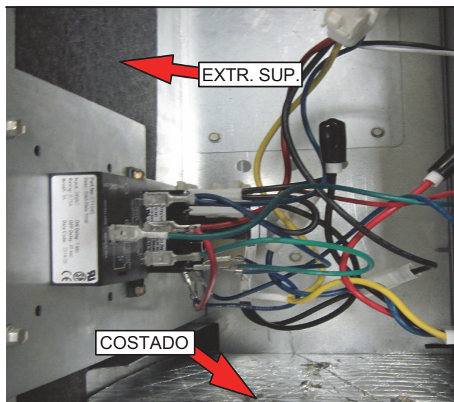
FIGURA 16. Panel de control reubicado al panel extremo (configuración horizontal izquierda)
