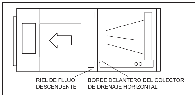
FIGURA 9. Configuración de descarga a la izquierda
