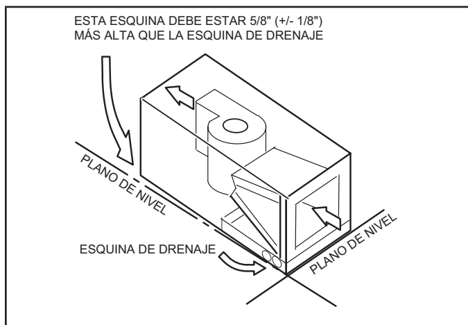
FIGURA 11. Inclinación de la unidad para un drenaje apropiado
