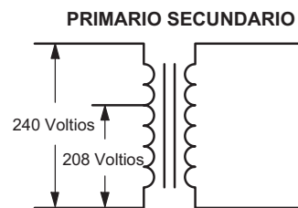
FIGURA 17. Conversión de la unidad de 240 VCA a 208 VCA
