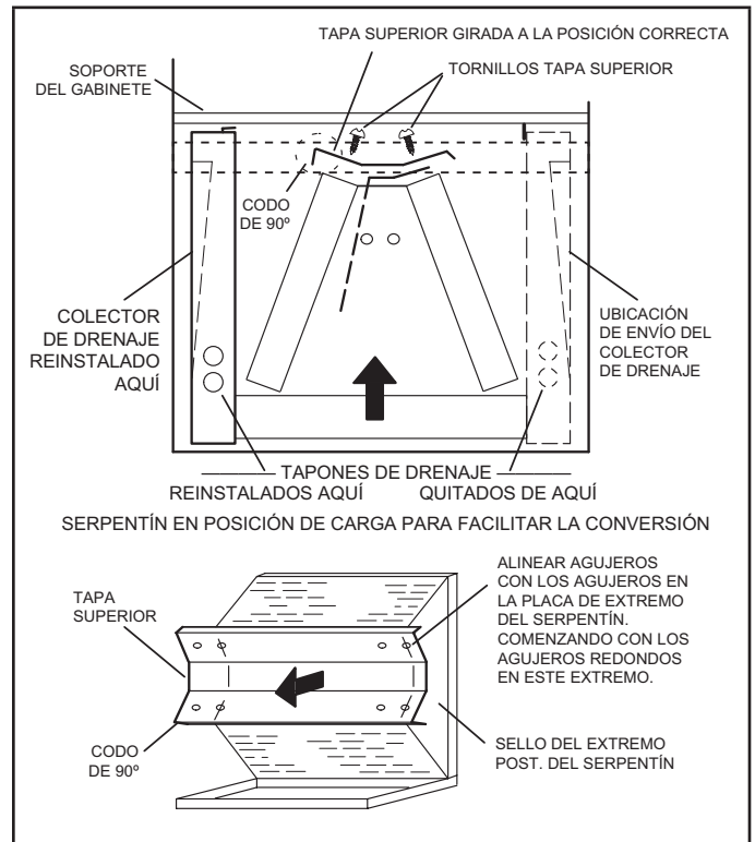
FIGURA 8. Modificación en el sitio para la descarga a la izquierda
