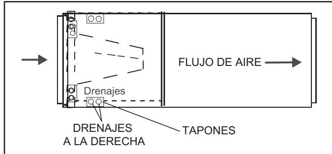
FIGURA 6. Configuración de descarga a la derecha
