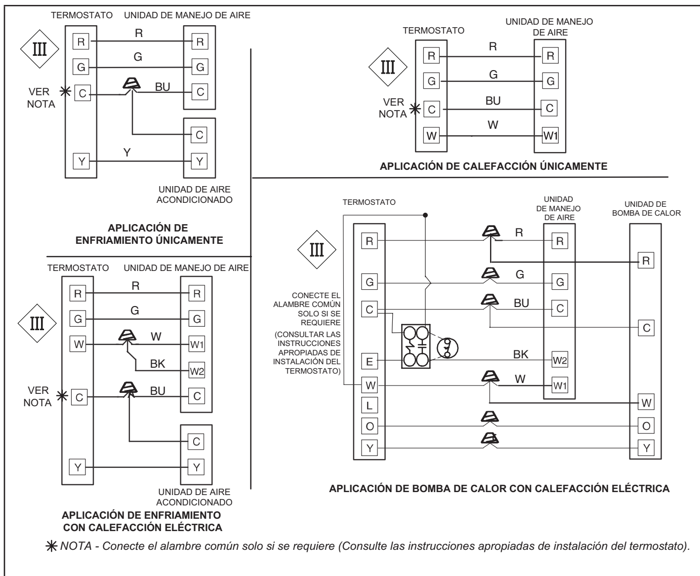
FIGURA 2. Conexiones de bajo voltaje (motor PSC de 3 velocidades): cableado en el sitio
