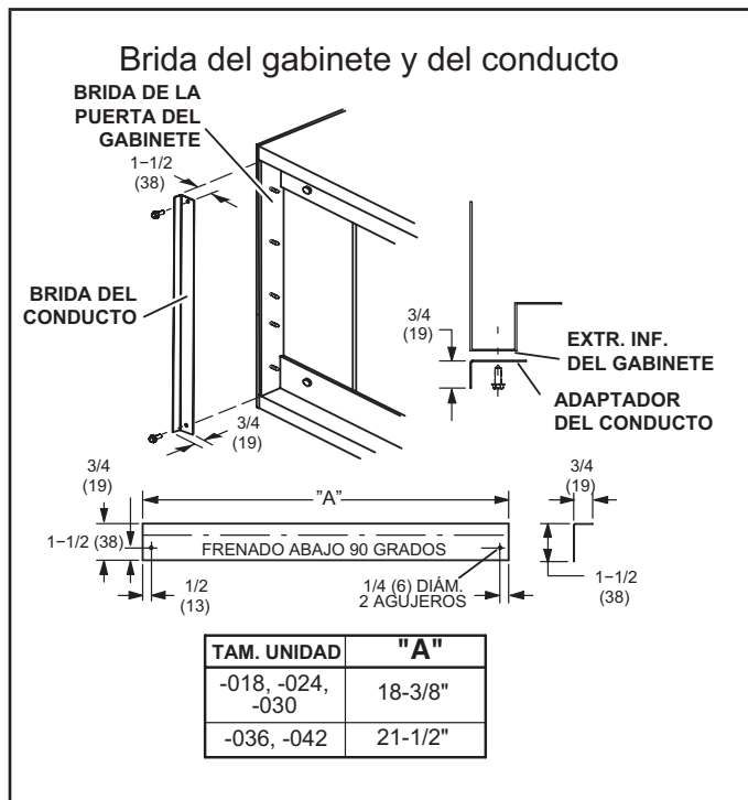
FIGURA 13. Brida del gabinete y del conducto
