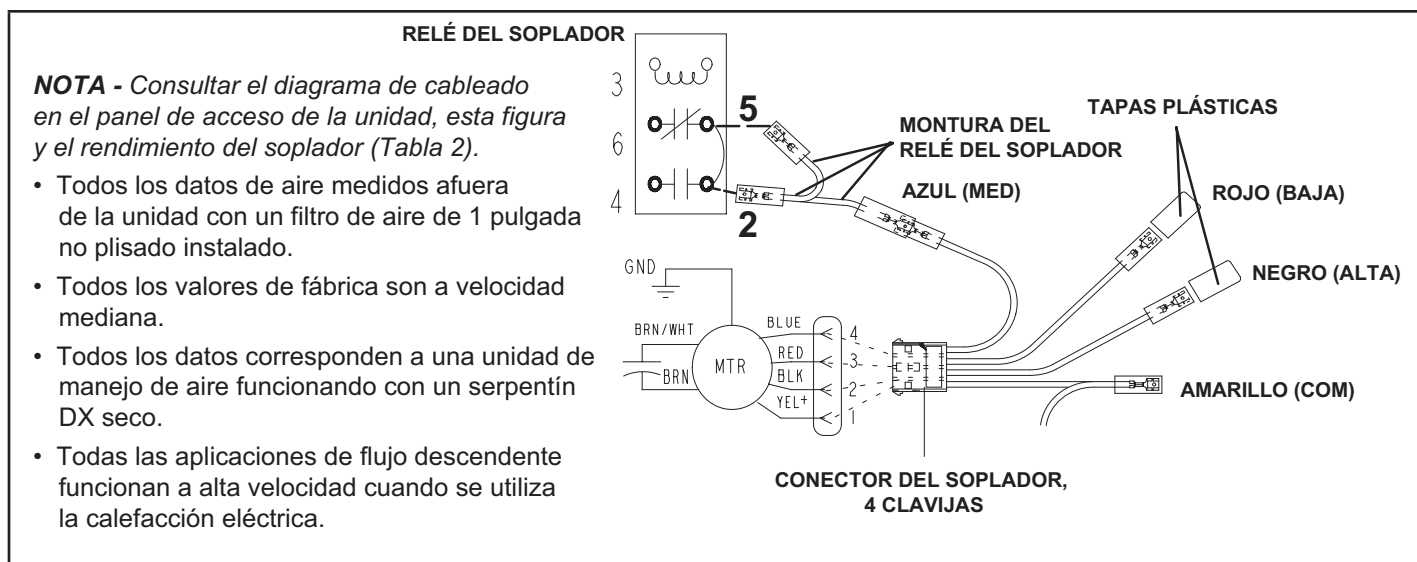
FIGURA 3. Cambio de velocidad del soplador
