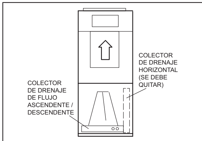
FIGURA 5. Configuración de flujo ascendente
