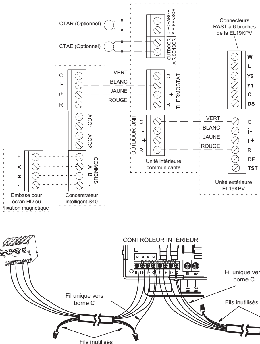
FIGURE 13. EL19KPV avec thermostat communicant S40 - Schéma de câblage sur place
