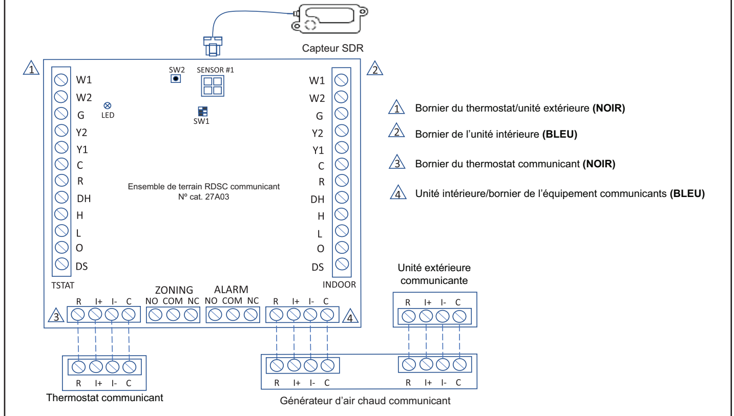
FIGURE 16. EL18KCV avec thermostat communicant S40 - Schéma de câblage sur place avec contrôleur du SDR
