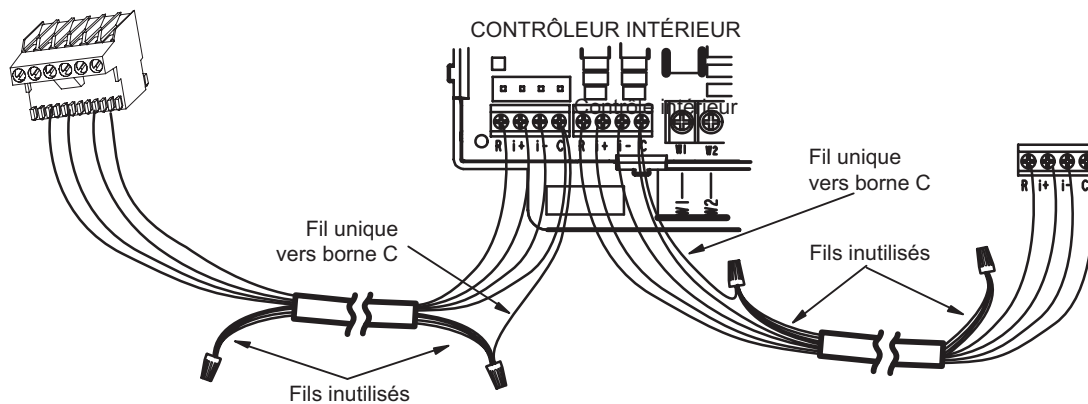
FIGURE 13. EL18KCV avec thermostat communicant S40 - Schéma de câblage sur place
