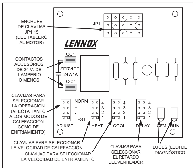
FIGURA 3. Selecciones de control de velocidad variable BDC3
