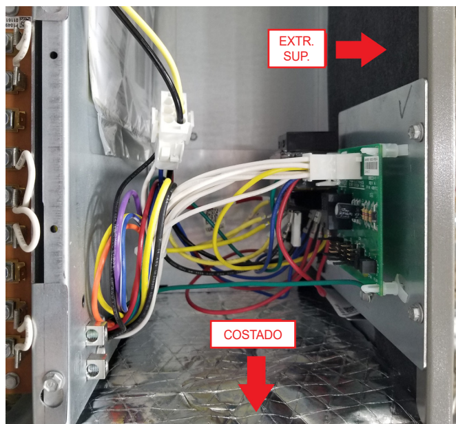
FIGURA 19. Panel de control reubicado al panel del extremo (configuración horizontal derecha)
