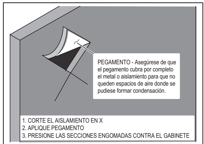
FIGURA 21. Reparación del aislamiento
