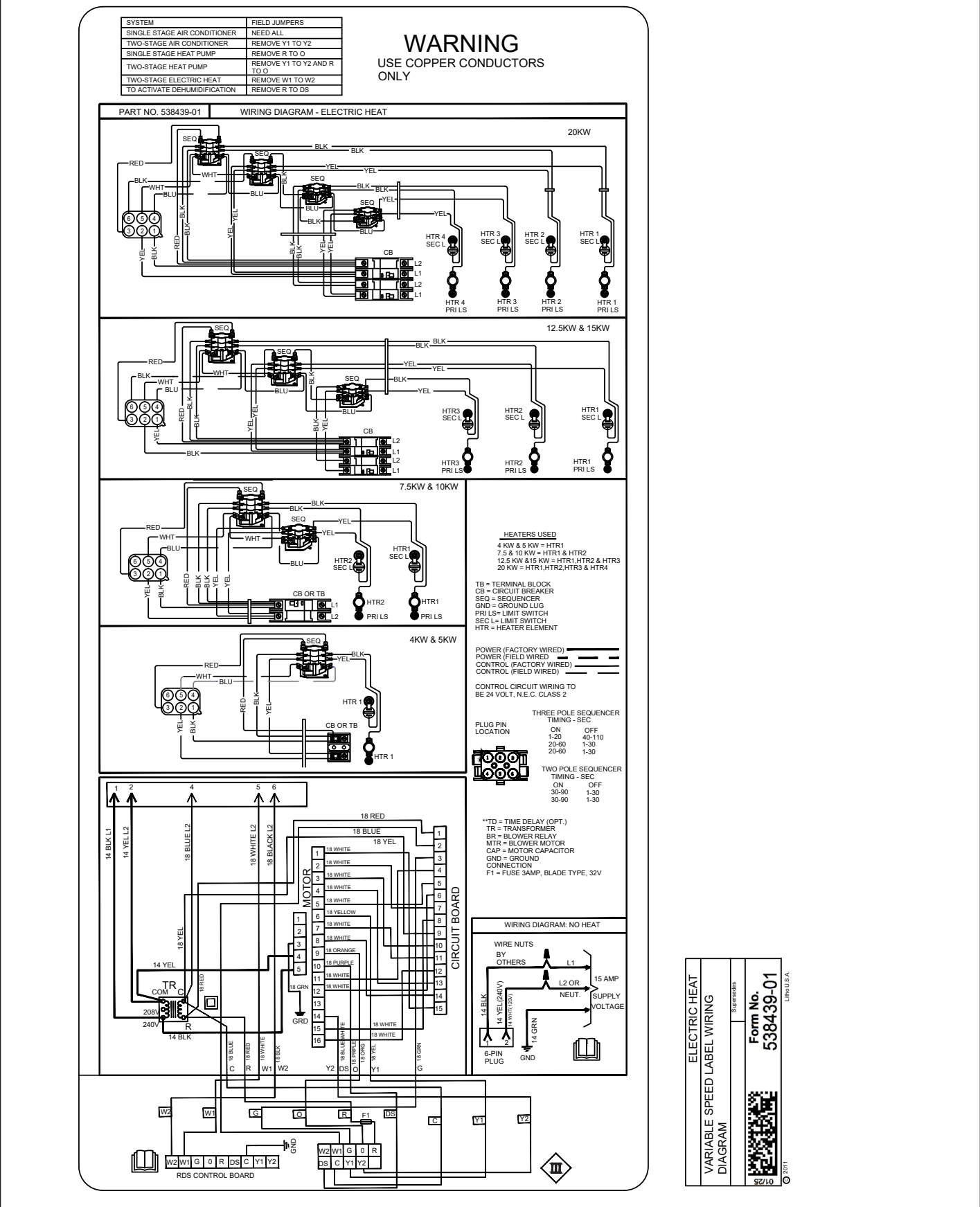
FIGURA 1. Diagrama de cableado típico, unidad de manejo de aire CBK45UHVT con calefacción eléctrica, (motor de velocidad variable)
