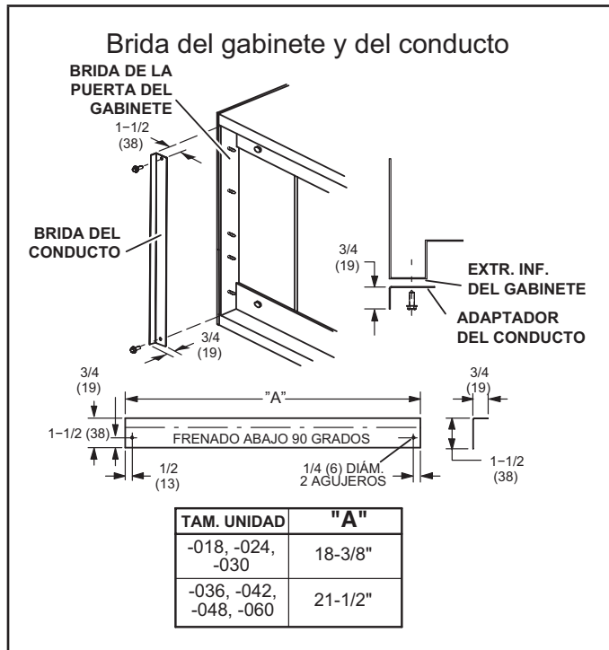
FIGURA 16. Brida del gabinete y del conducto
