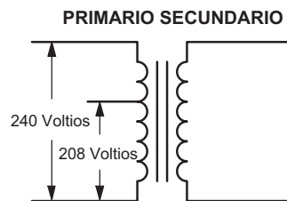
FIGURA 20. Conversión de la unidad de 240 VCA a 208 VCA
