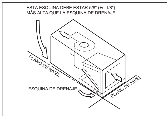
FIGURA 14. Inclinación de la unidad para un drenaje apropiado
