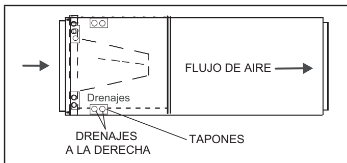
FIGURA 5. Configuración de descarga a la derecha
