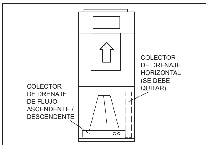
FIGURA 4. Configuración de flujo ascendente
