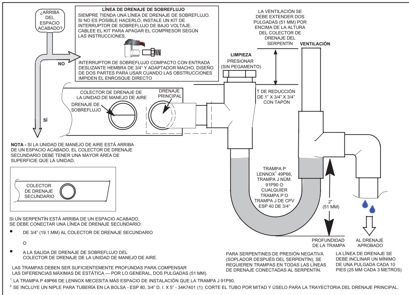
FIGURA 13. Drenaje típico principal y de sobreflujo
