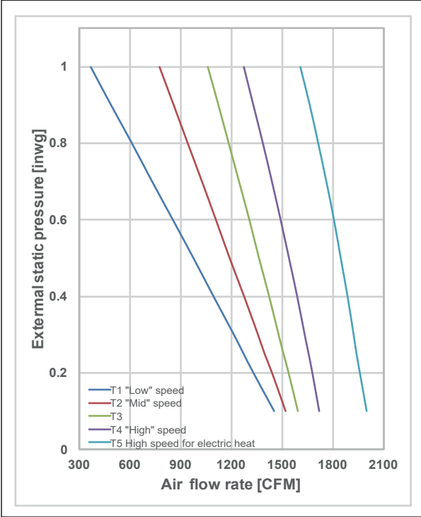
7) VVCC054S4-4P
