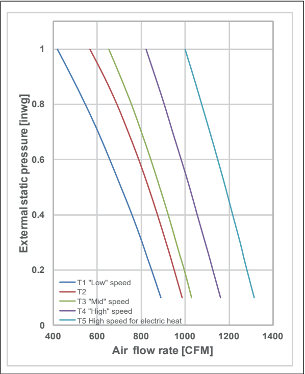
5) VVCC036S4-4P
