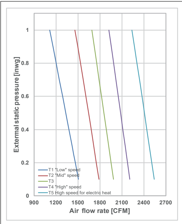
9) VVCC072S4-4P
