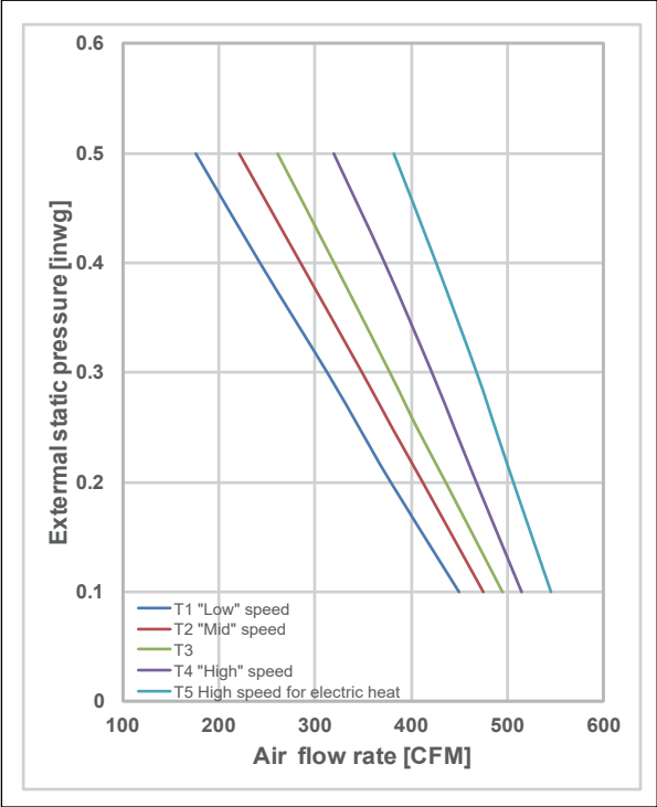
1) VVCC012S4-4P
