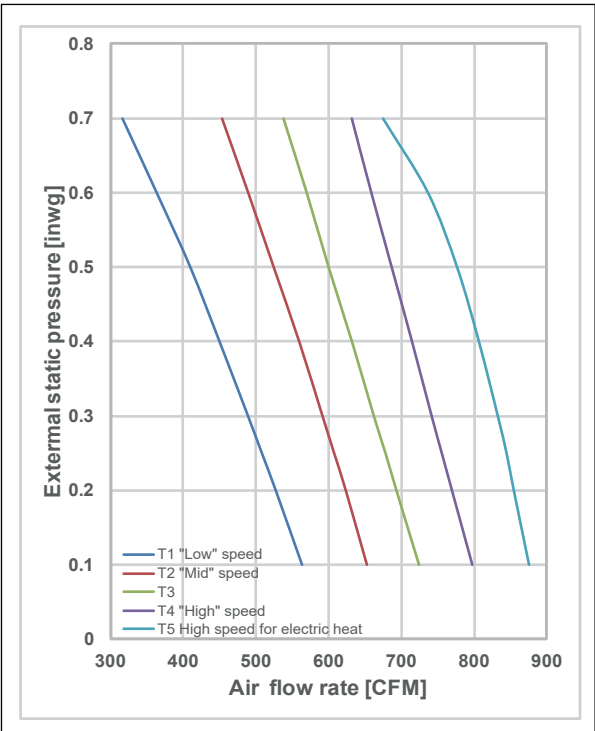
3) VVCC024S4-4P
