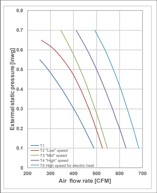
2) VVCC018S4-4P
