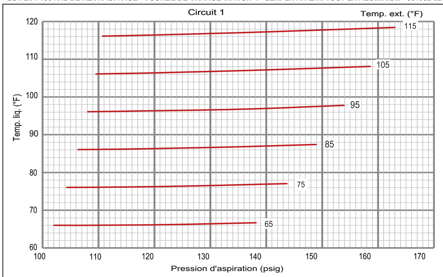
LGT/LCT 156 PAS DE RÉCHAUFFAGE - COURBE DE CHARGE CIRCUIT 1 - SERPENTIN EXT. TOUT EN ALUMINIUM - 581082-02
