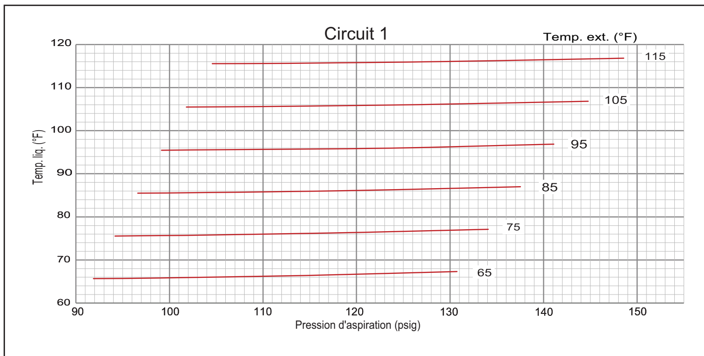
LGT/LCT 180 PAS DE RÉCHAUFFAGE - COURBE DE CHARGE CIRCUIT 1 - SERPENTIN EXT. TOUT EN ALUMINIUM - 581086-02
