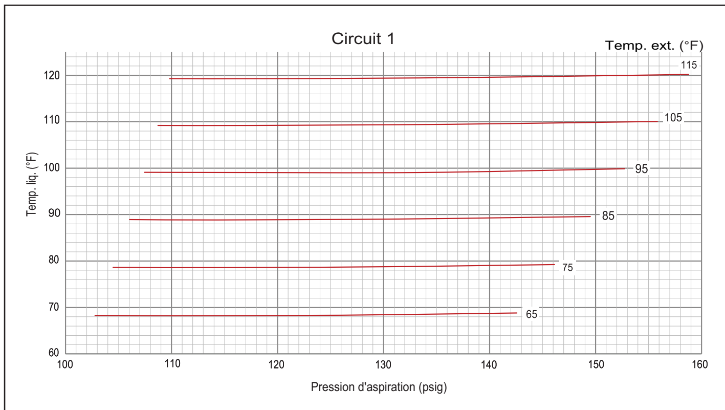
LGT/LCT 300 RÉCHAUFFAGE - COURBE DE CHARGE CIRCUIT 1 - SERPENTIN EXT. TOUT EN ALUMINIUM - 581100-02
