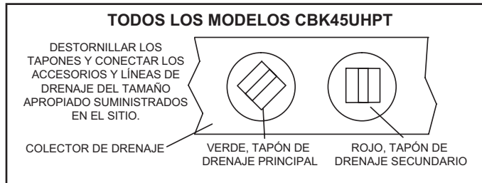
FIGURA 15. Conexiones de las líneas de drenaje
