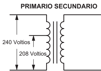
FIGURA 18. Conversión de la unidad de 240 VCA a 208 VCA
