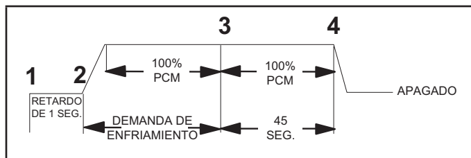
FIGURA 19. Retardo de tiempo del soplador
