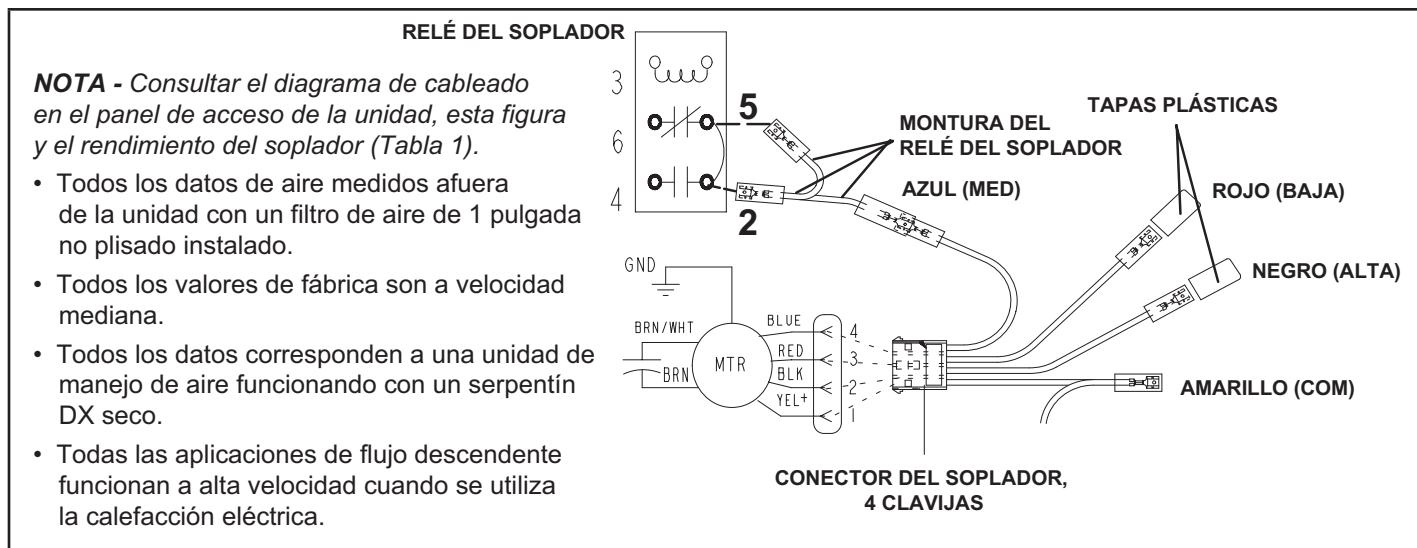
FIGURA 3. Cambio de velocidad del soplador
