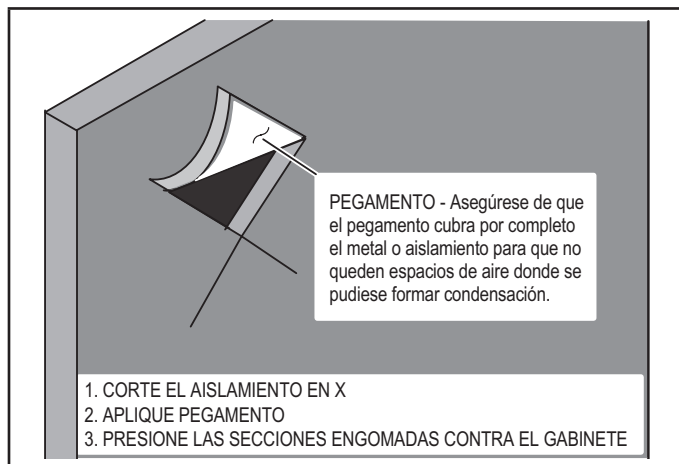
FIGURA 20. Reparación del aislamiento
