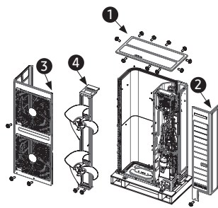
〈UB4 - Outdoor unit〉
