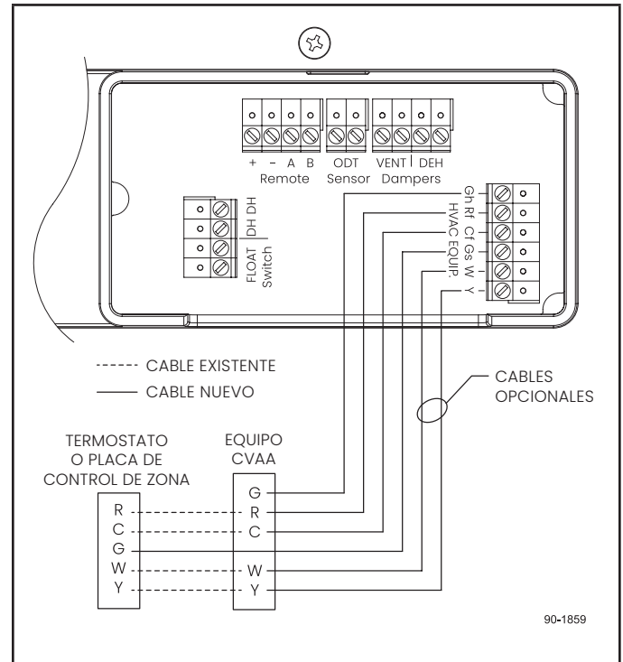
Figura 24. Cableado al sistema de CVAA
