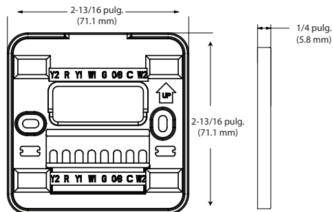
Figura 1. Termostato, cubierta y placa posterior del Lennox M40
