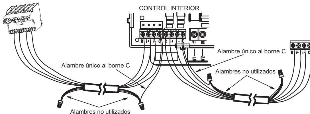
FIGURA 13. EL18KCV con termostato S40 con comunicación – Diagrama de cableado en el sitio
