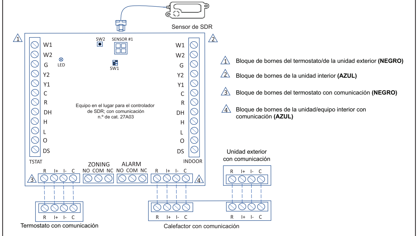
FIGURA 16. Diagrama de cableado en el sitio con controlador SDR para el sistema EL18KCV con termostato S40 con comunicación.
