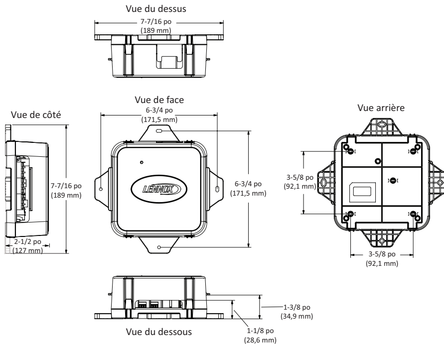
Figure 2. Contrôleur communicant pour SDR - Dimensions
