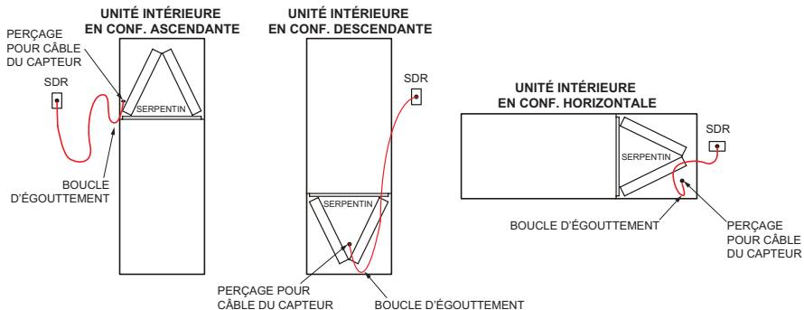
Figure 3. Acheminement du câble du capteur
