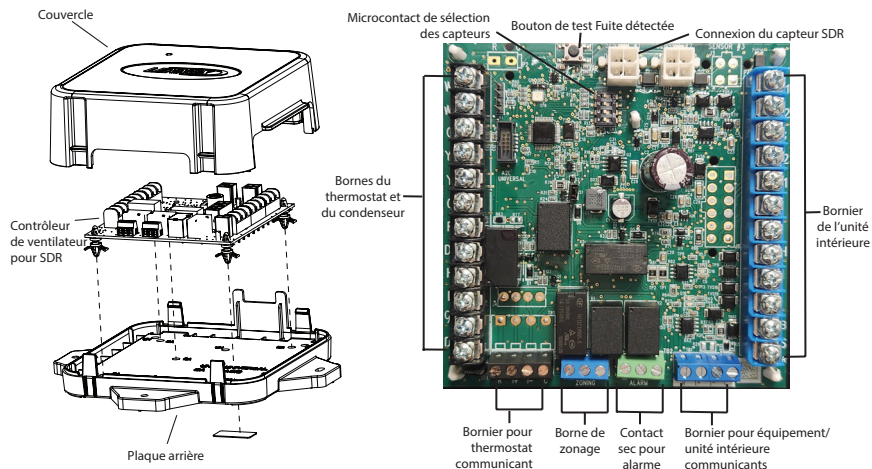
Figure 1. Contrôleur communicant pour SDR
