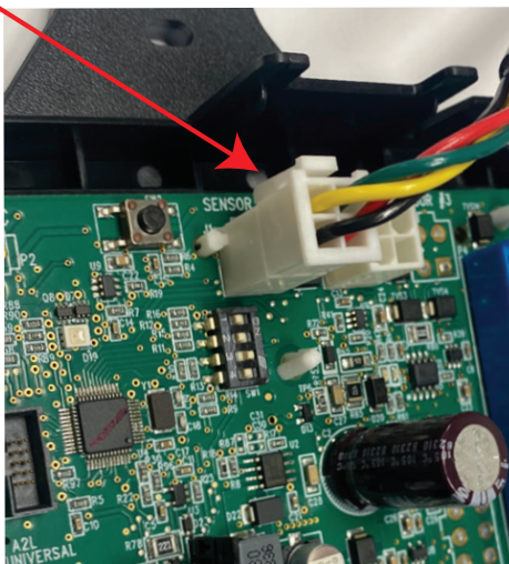
Figure 4. Raccordement du capteur SDR au contrôleur de ventilateur pour SDR
