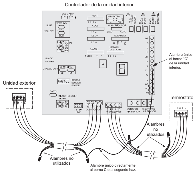
Figura 13. Reducción al mínimo del ruido eléctrico
