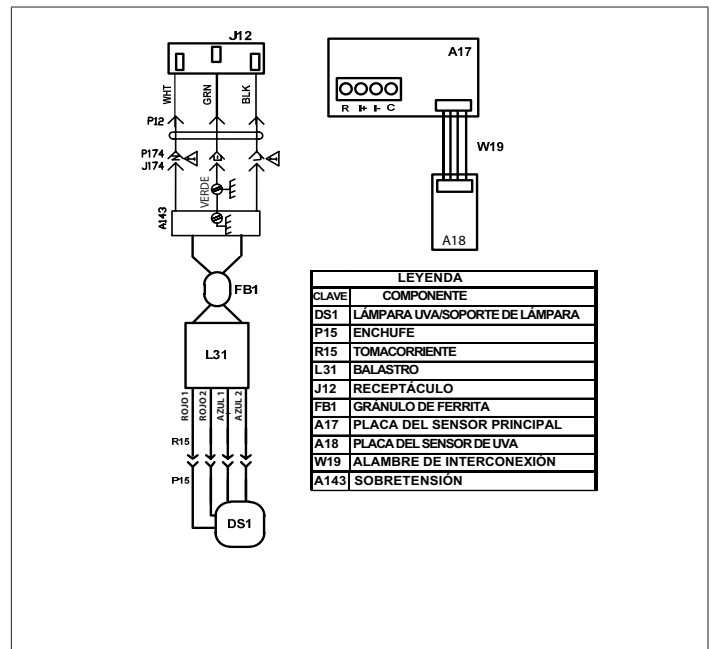
Figura 15. Diagrama esquemático de cableado del PCO
