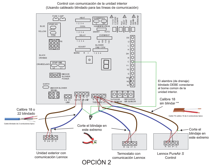
Figura 11. Conexiones de cableado del sistema con comunicación Lennox (Opción 2)
