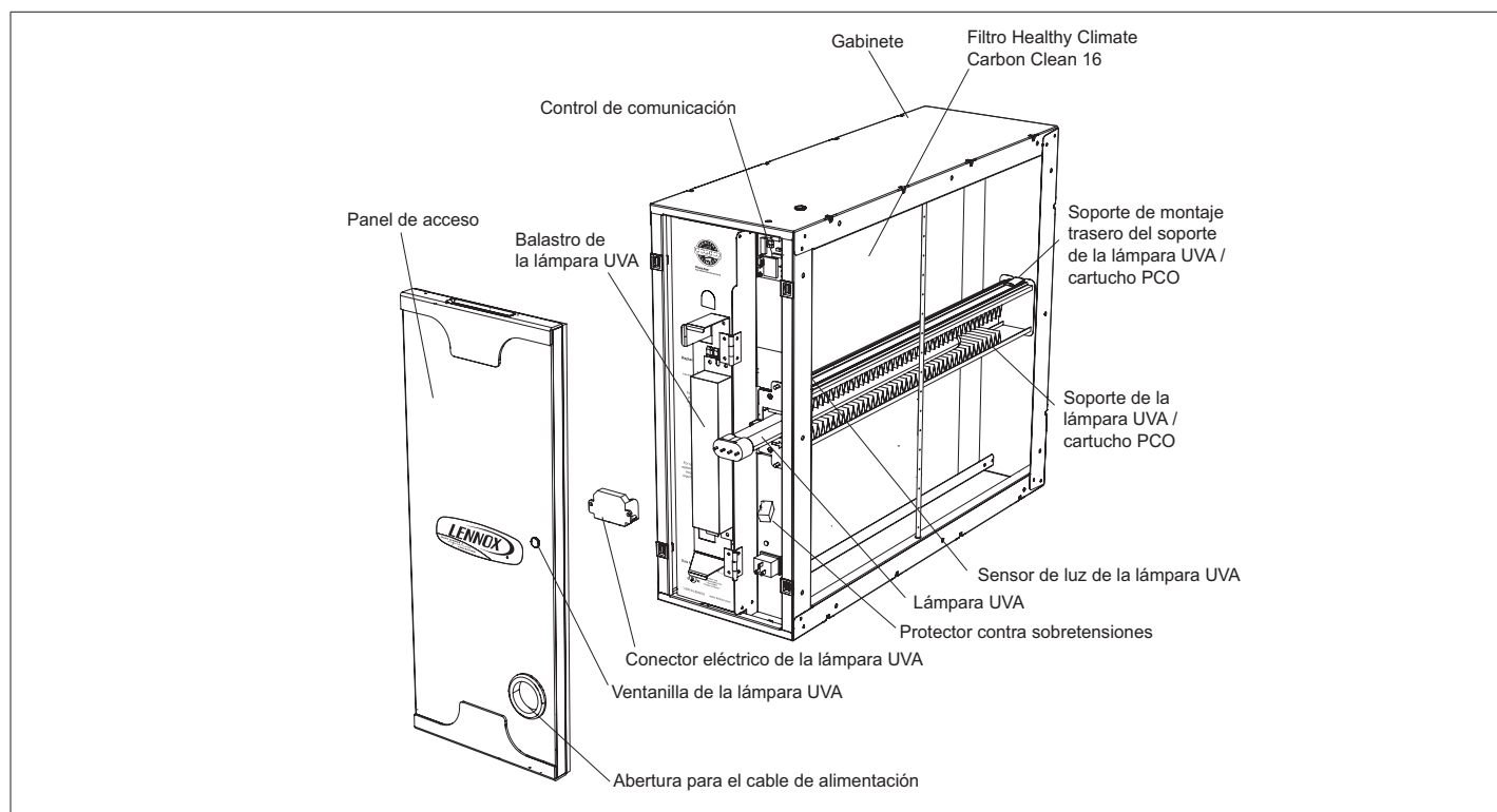
Figura 1. Identificación de partes
