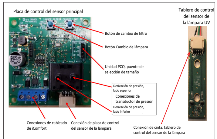
Figura 16. Control de comunicación de PureAir S
