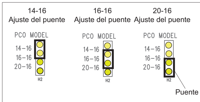
Figura 17. Selección de puente del modelo
