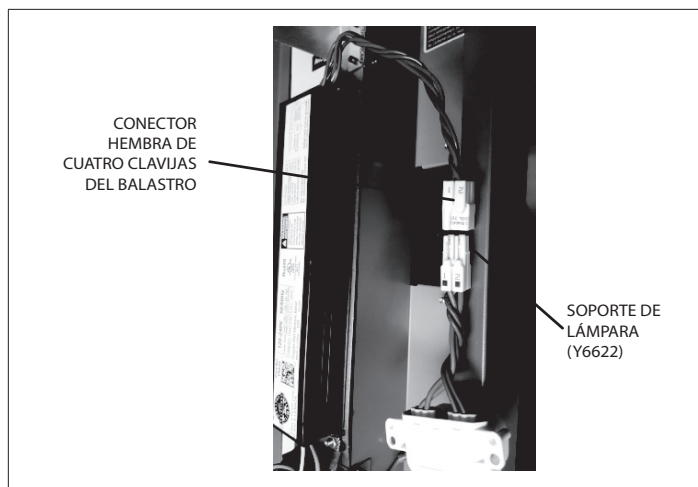
Figura 9. Conector hembra de 4 clavijas del balastro
