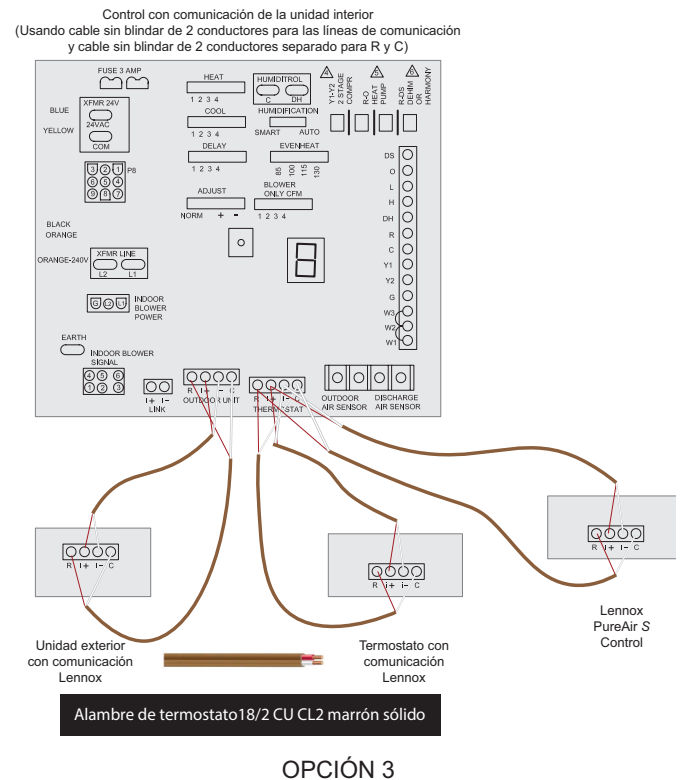
Figura 12. Conexiones de cableado del sistema con comunicación Lennox usando cable sin blindar separado (Opción 3)
