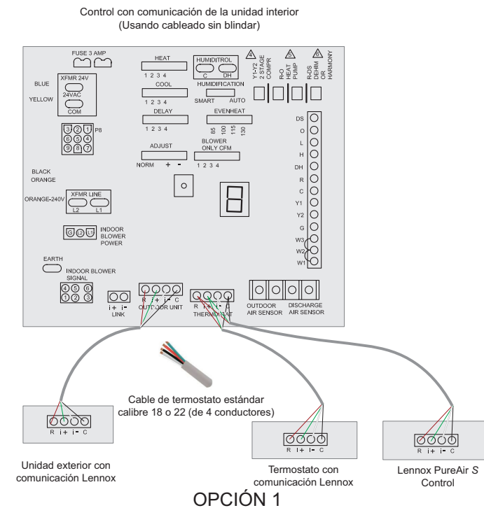
Figura 10. Conexiones de cableado del sistema con comunicación Lennox (Opción 1)
