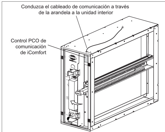
Figura 14. Ruta del cableado de comunicación
