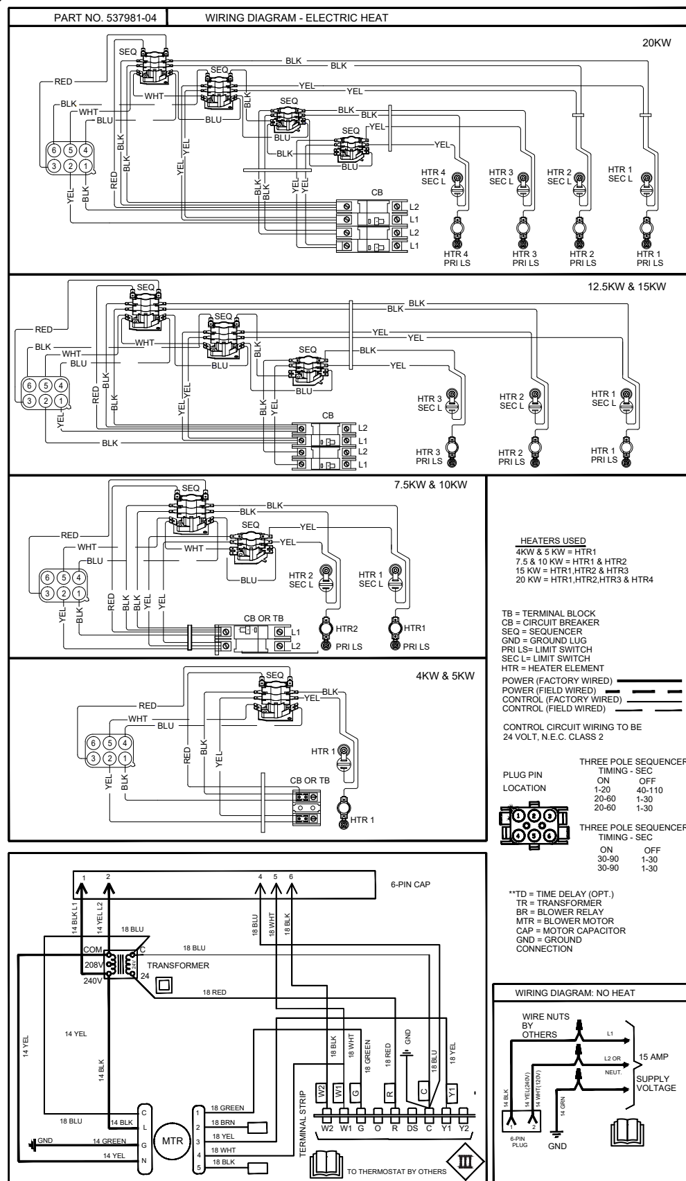
FIGURA 1. Diagrama de cableado típico – Unidad de manejo de aire CBA25UHE con calefacción eléctrica – CT
