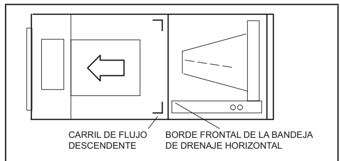
FIGURA 11. Configuración de descarga a la izquierda
