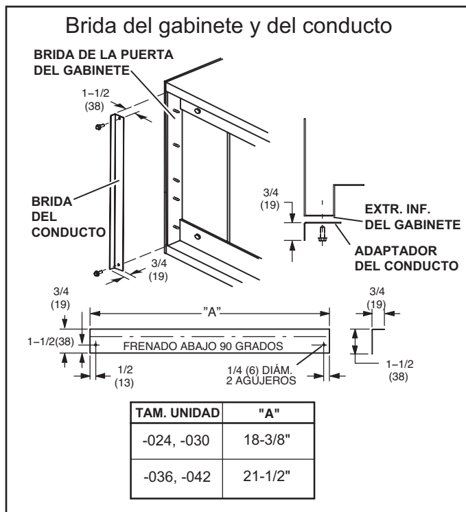
FIGURA 15. Brida del gabinete y del conducto
