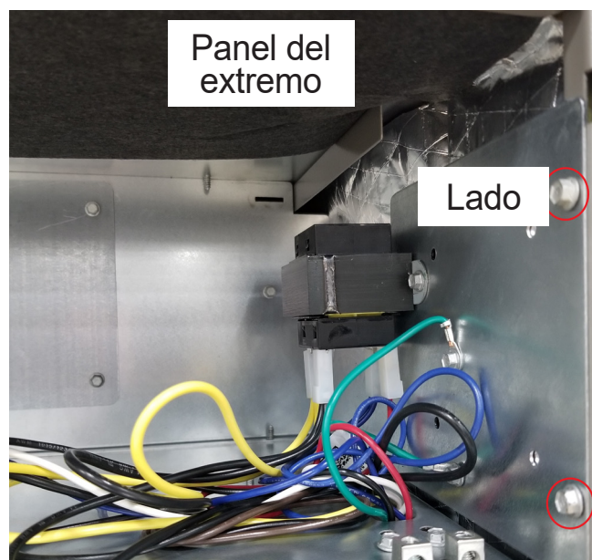
FIGURA 3. Conexiones eléctricas (configuración de flujo ascendente)
