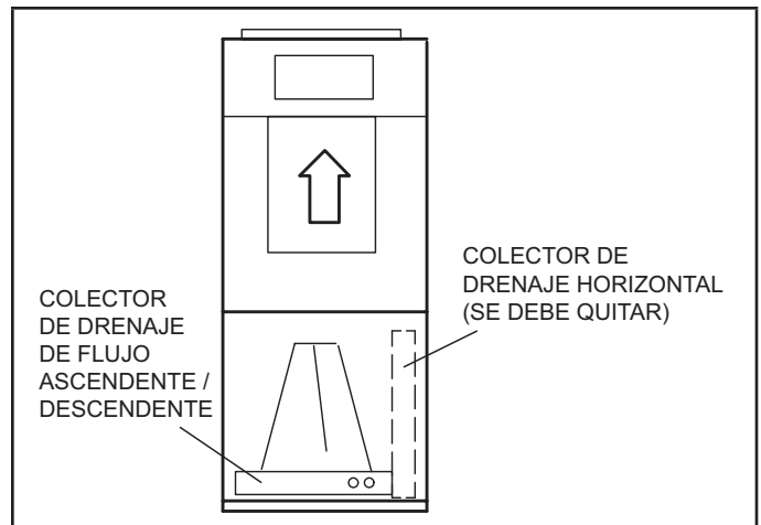
FIGURA 7. Configuración de flujo ascendente APLICACIONES HORIZONTALES
