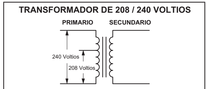
FIGURA 6. Conversión de la unidad de 240 VCA a 208 VCA
