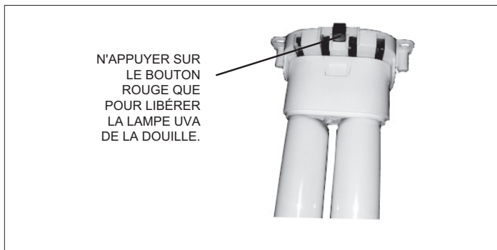
Figure 5. Libération de la lampe UVA de la douille
