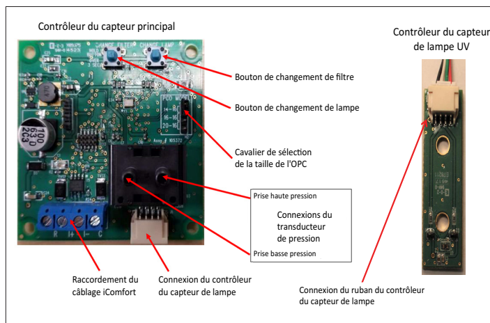
Figure 16. Contrôleur communicant du PureAir S
