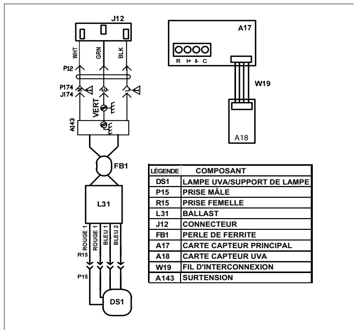
Figure 15. Schéma de câblage de la cartouche OPC
