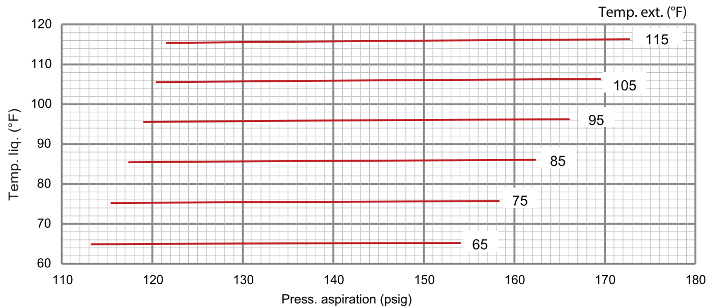
036 Courbe de charge - Réchauffage - Serpentin tout en aluminium - 581267-01
