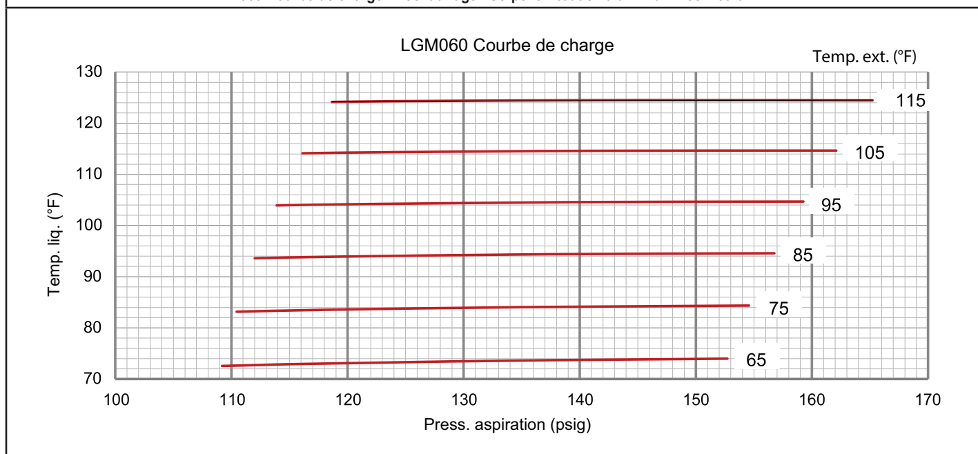
060 Courbe de charge - Réchauffage - Serpentin tout en aluminium - 581269-01
