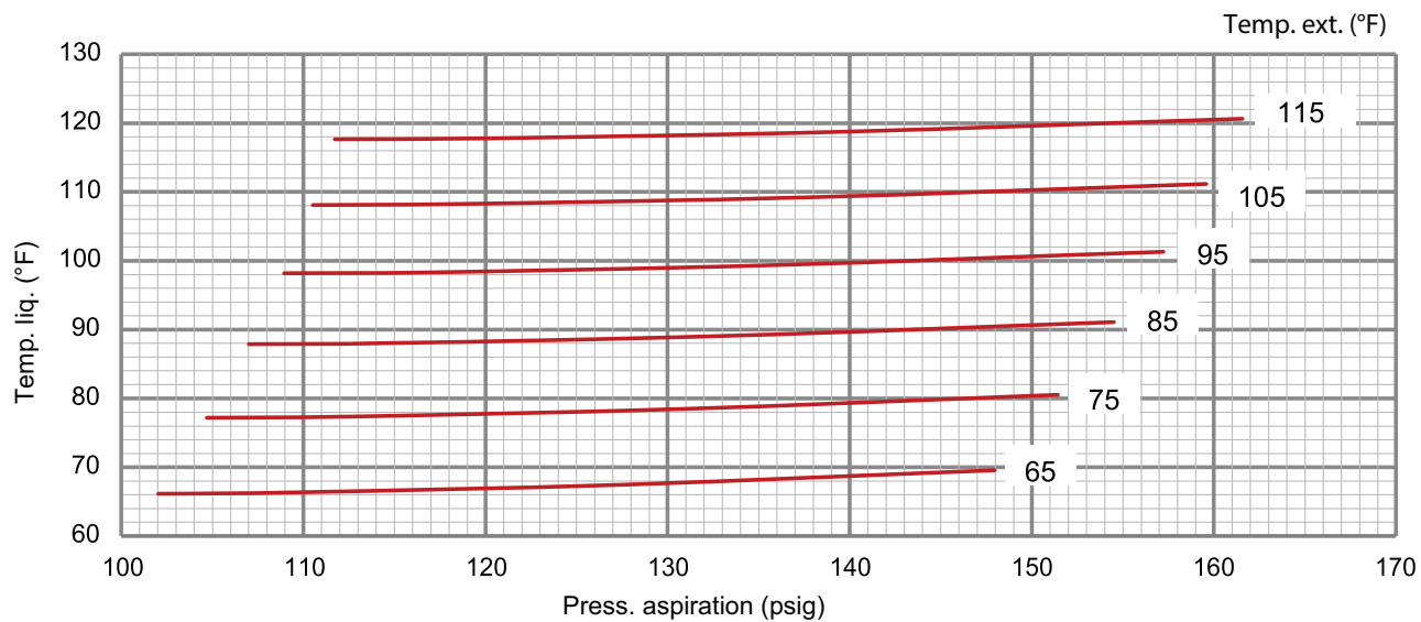
074 Courbe de charge - Réchauffage - Serpentin tout en aluminium - 581270-01
