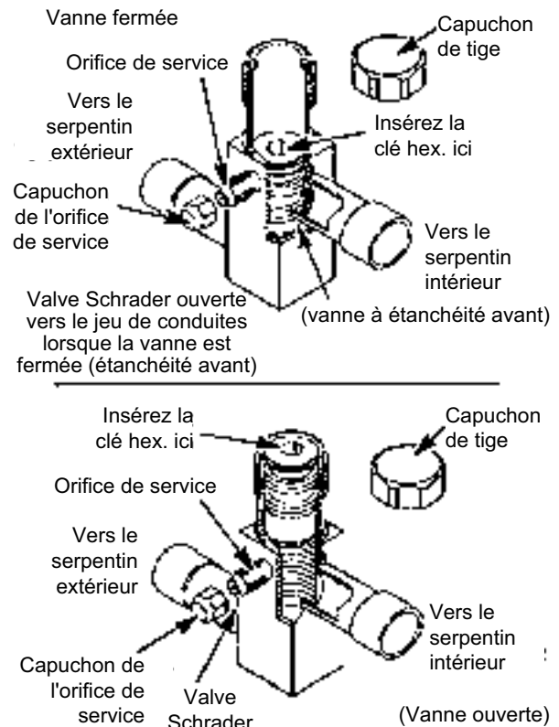
FIGURE 14. Fonctionnement de la vanne de service d'angle
