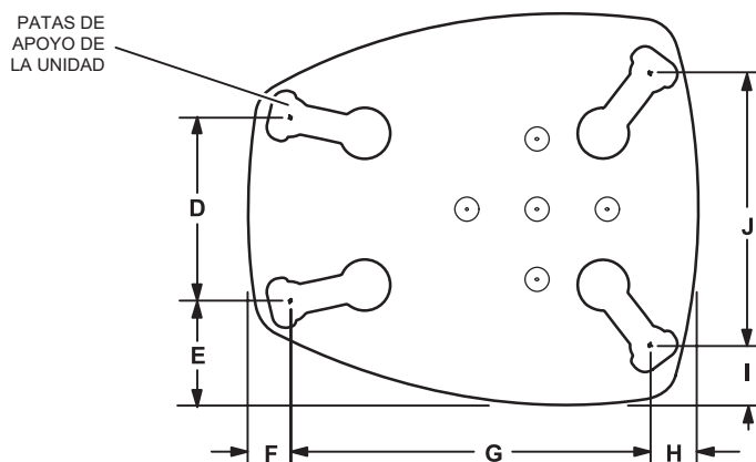
BASE DE EL15KC1-030 A -060 CON SOPORTES ALARGADOS
