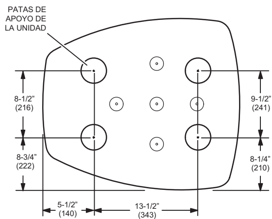
SECCIÓN DE LA BASE DE EL15KC1-018 Y EL15KC1-024 (PEQUEÑA)
