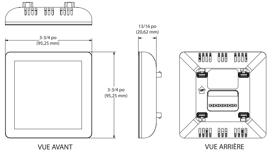
Figure 2. Dimensions du thermostat
