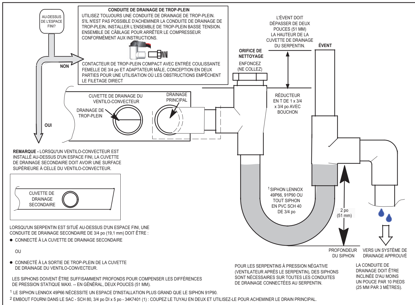
FIGURE 12. Drain principal et drain de trop-plein types
