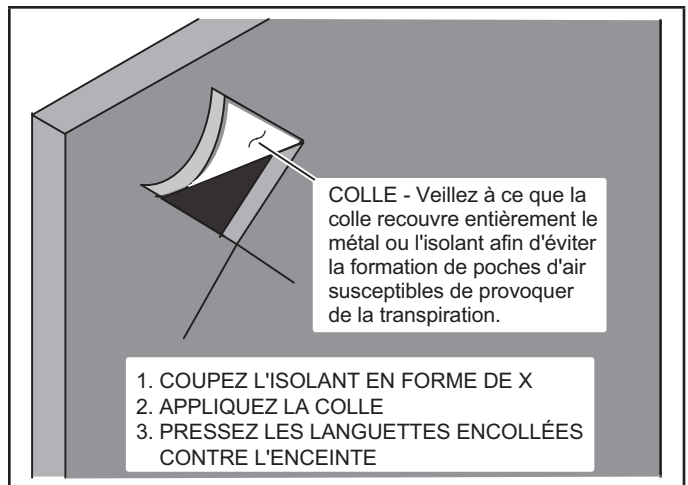
FIGURE 21. Réparation de l'isolation
