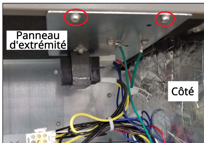
FIGURE 19. Panneau du contrôleur déplacé vers le panneau d'extrémité (Configuration horizontale avec refoulement par la droite)
