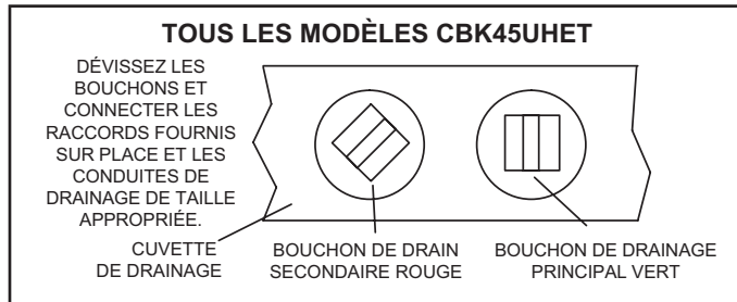
FIGURE 14. Connexions des conduites de drainage
