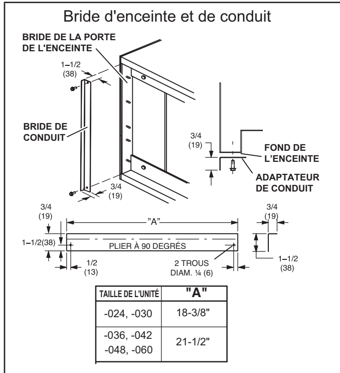
FIGURE 15. Bride d'enceinte et de conduit
