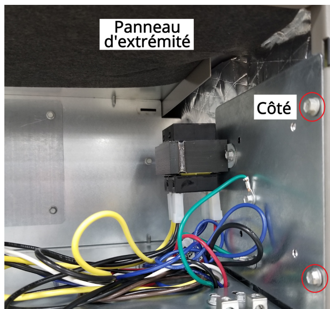
FIGURE 17. Connexions électriques (Configuration ascendante)
