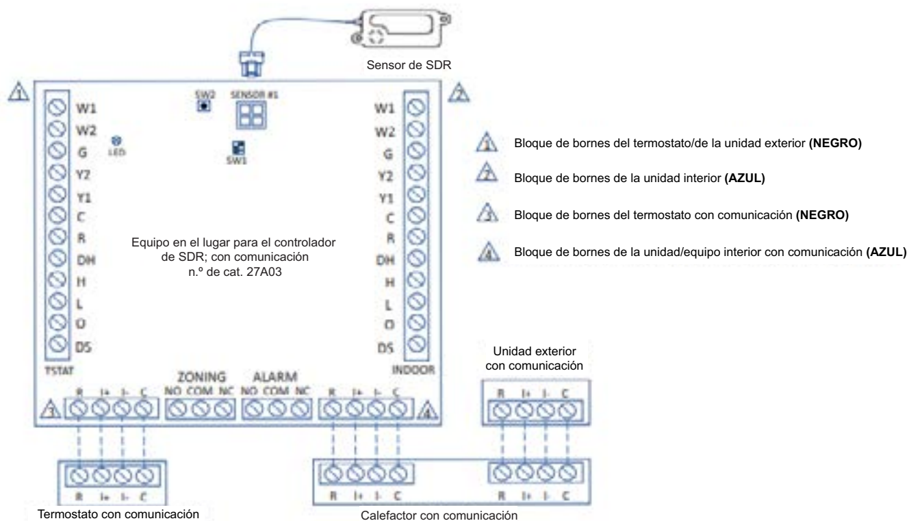
FIGURA 12. Diagrama de cableado en el sitio con controlador SDR para el sistema SL25KCV con termostato S40 con comunicación
