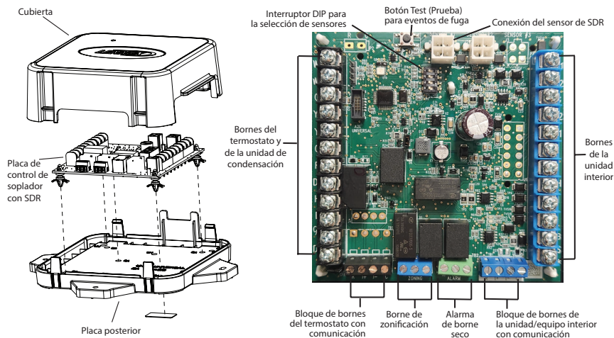
Figura 1. Placa de control con comunicación con SDR
