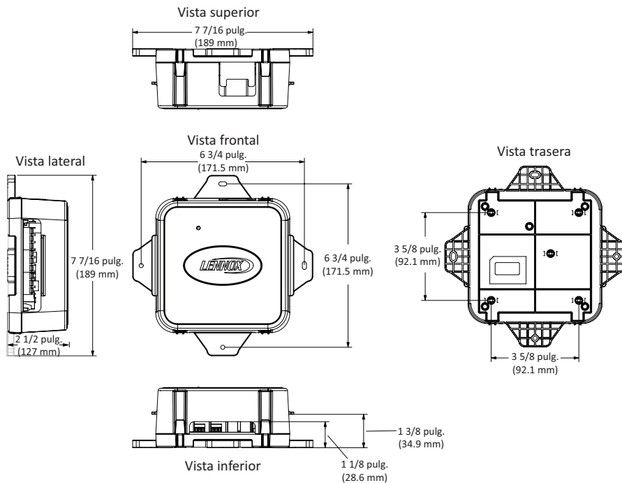
Figura 2. Dimensiones de la placa de control con comunicación con SDR
