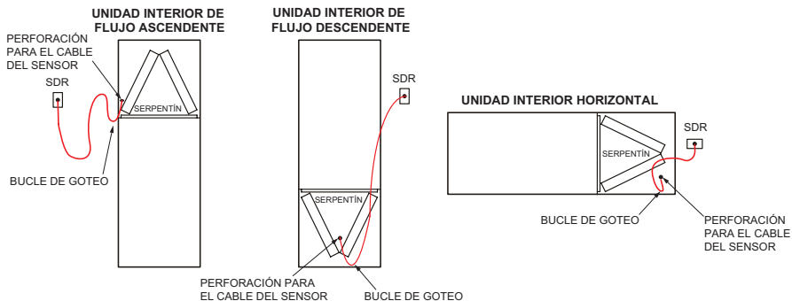
Figura 3. Cableado del sensor
