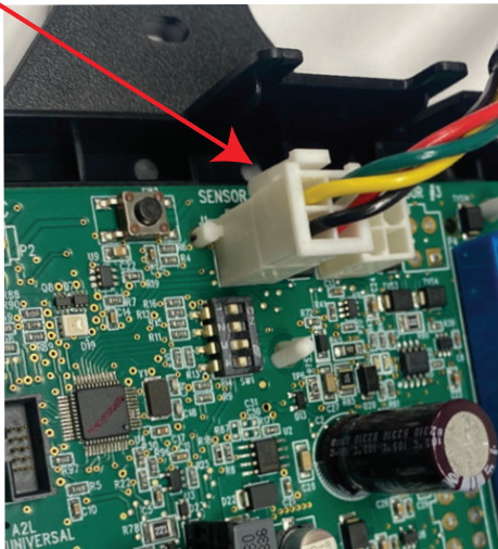
Figura 4. Conexión del sensor del SDR a la placa de control del soplador con SDR
