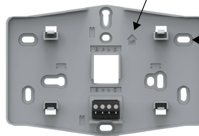
Base secundaria del termostato (Vista frontal)
