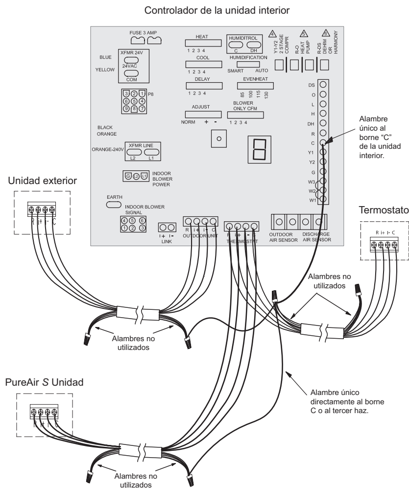
Figura 13. Cable de termostato sin blindar (conductores múltiples) utilizado para cablear la unidad interior con comunicación a PureAir S
