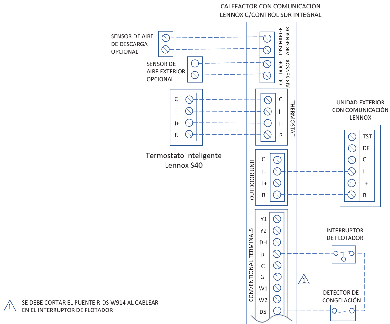
Figura 11. Kit de enclavamiento de S40 Lennox inteligente y filtro de desvío HEPA y humidificador
