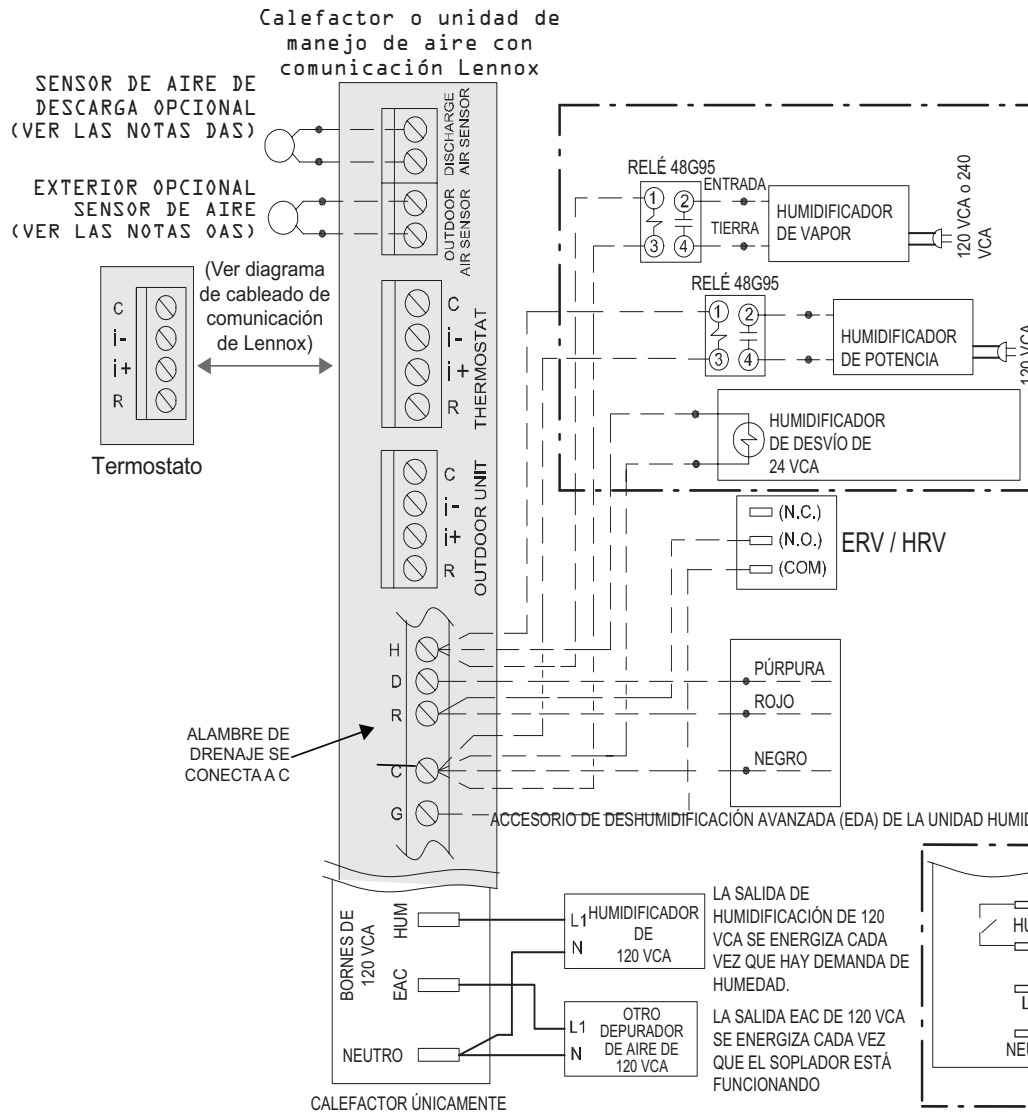
Figura 9. S40 Lennox inteligente con accesorio humidificador
