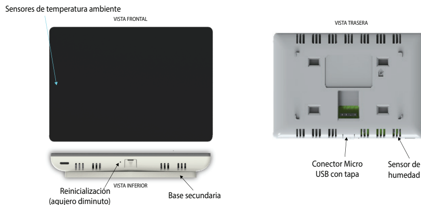
Figura 1. Componentes externos del termostato
