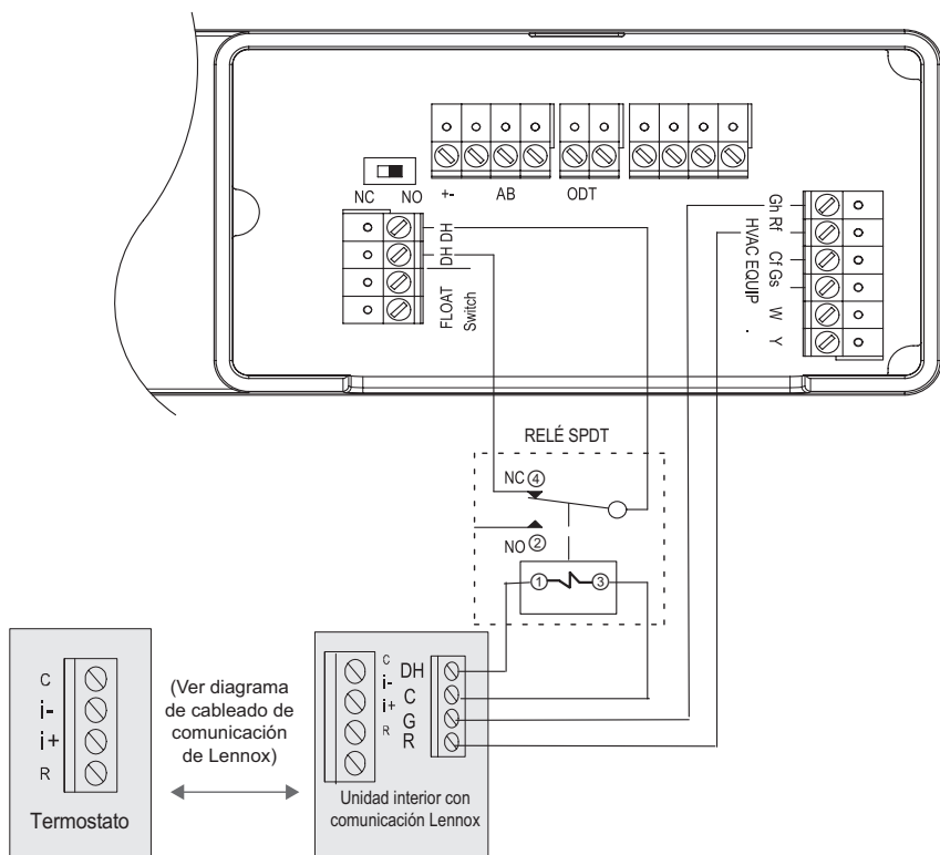
Figura 7. S40 Lennox inteligente, control interior con comunicación (conexiones convencionales), relé y deshumidificadores Serie HCWHD4
