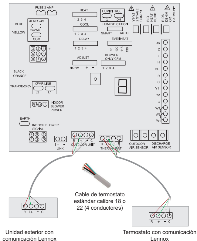
Figura 4. Conexiones de cableado del sistema con comunicación Lennox usando cable sin blindar (Opción 2) o blindado (Opción 3)
