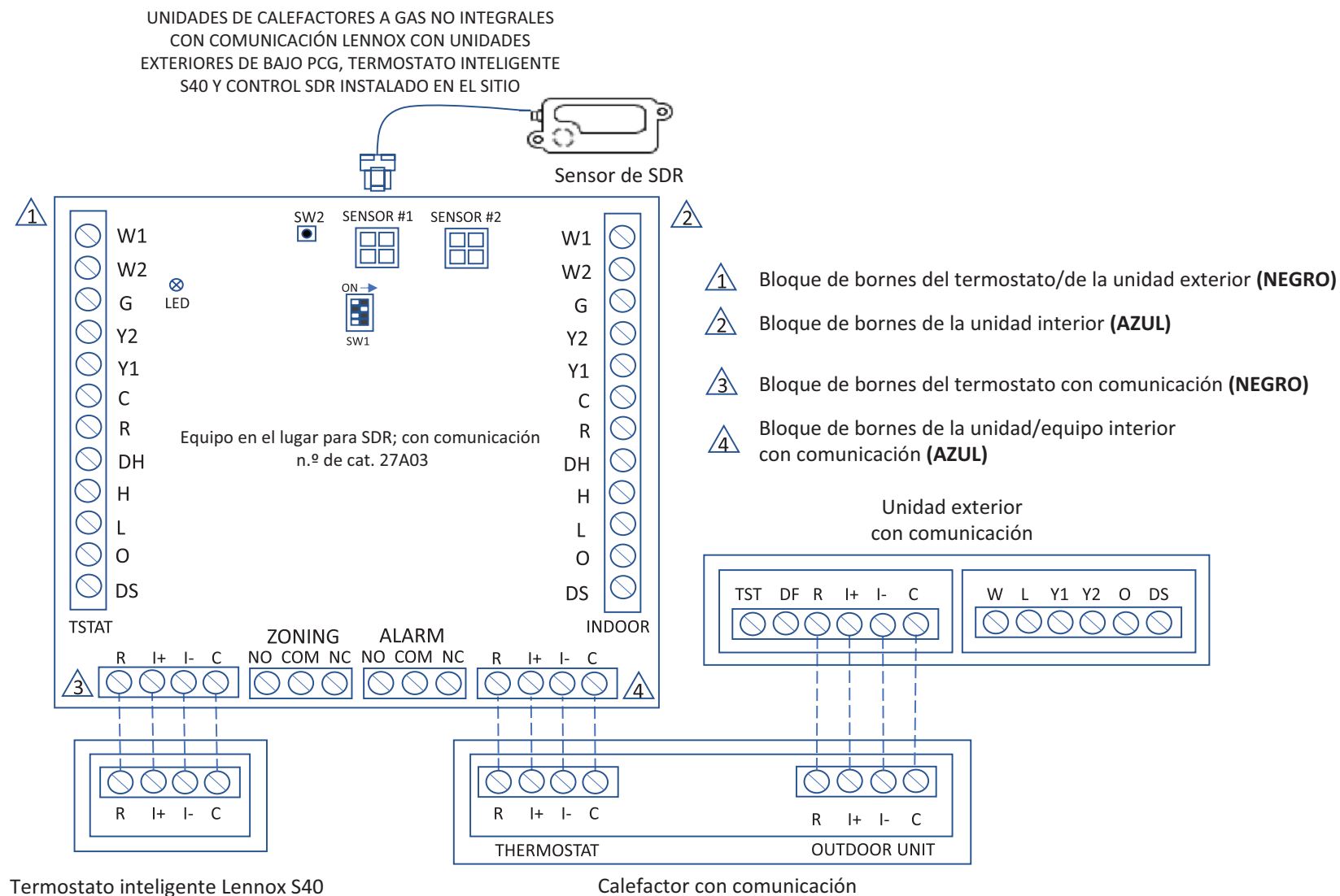
Figura 17. S40 Lennox inteligente, calefactor a gas con comunicación no integral con unidad exterior de bajo PCG y control RDS de Lennox
