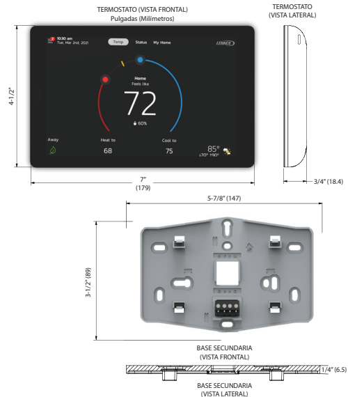
Figura 2. Termostato y base secundaria
