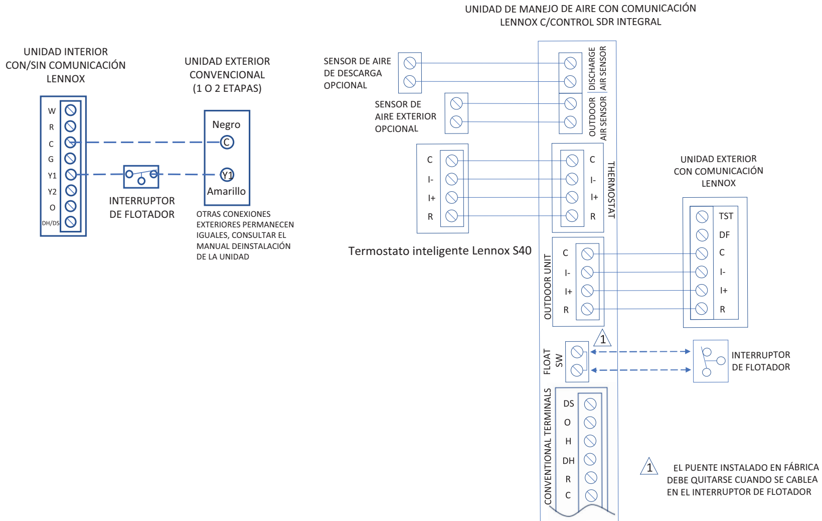
Figura 12. S40 Lennox inteligente, controles interiores con comunicación Lennox e interruptor de flotador
