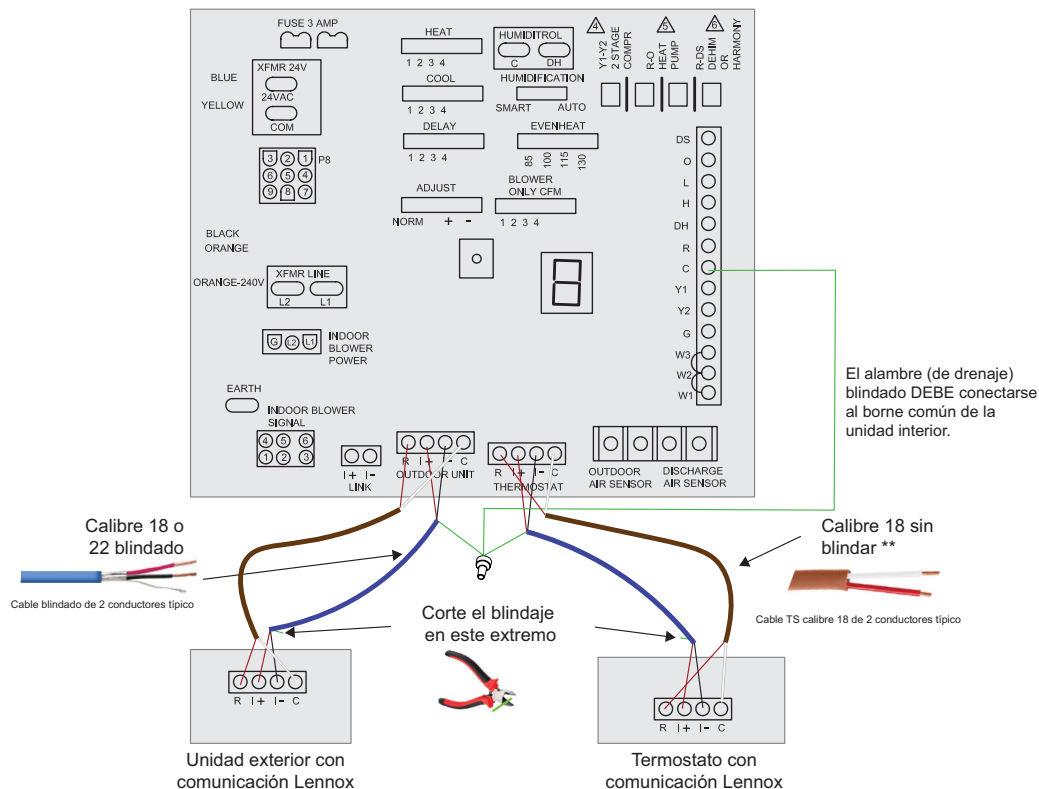
Figura 4. Conexiones de cableado del sistema con comunicación Lennox usando cable sin blindar (Opción 2) o blindado (Opción 3)
