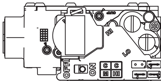
VANNE DE GAZ ILLUSTRÉE EN POSITION ON/OUVERTE
