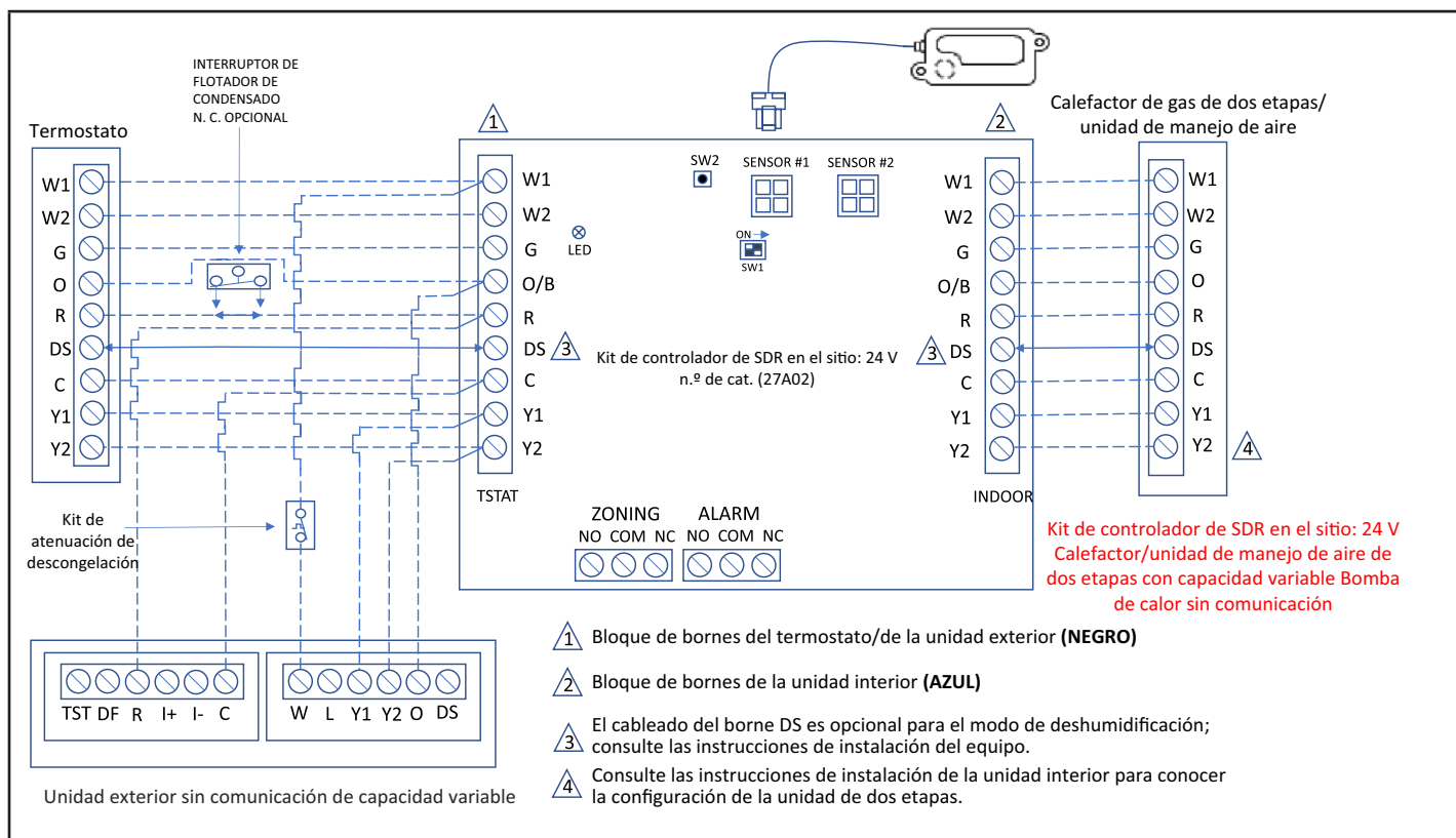
FIGURA 13. Termostato sin comunicación/Unidad exterior sin comunicación con controlador RDS
