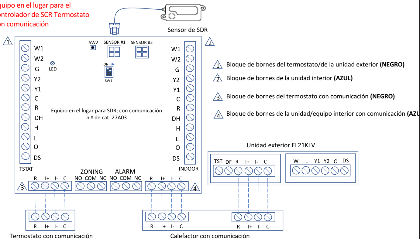
FIGURA 12. Termostato S40 con comunicación/Calefactor con comunicación con controlador RDS.
