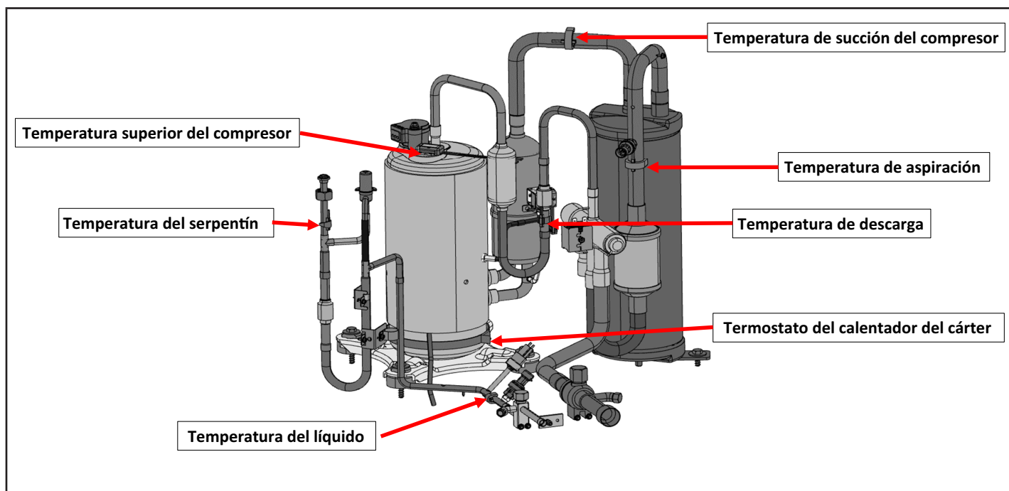
FIGURA 15. Ubicaciones del sensor de temperatura
