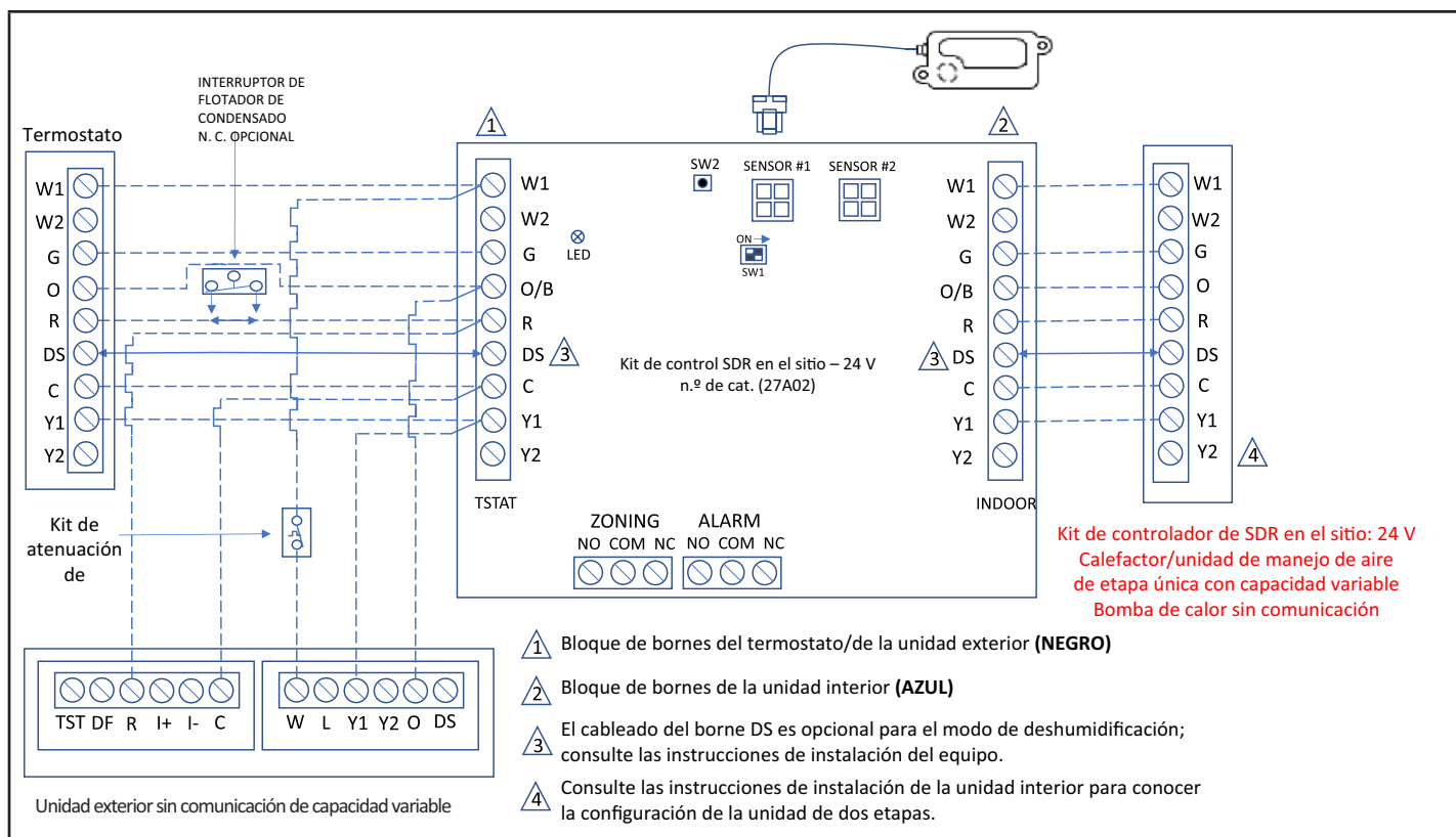
FIGURA 14. Termostato sin comunicación/Bomba de calor sin comunicación con controlador RDS
