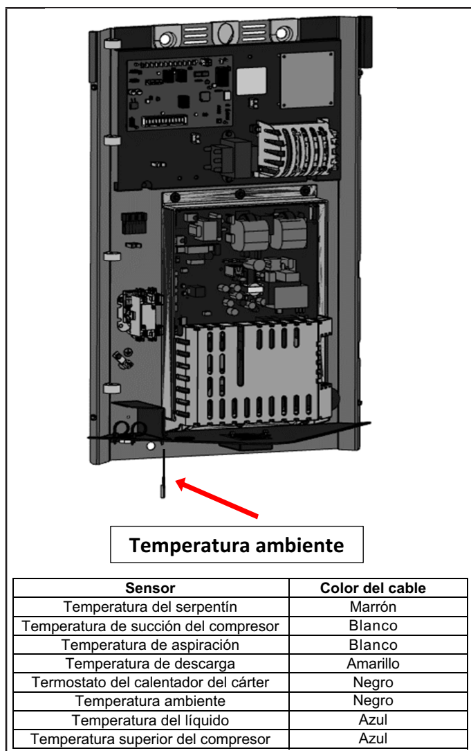
FIGURA 16. Ubicación del sensor/Cableado
